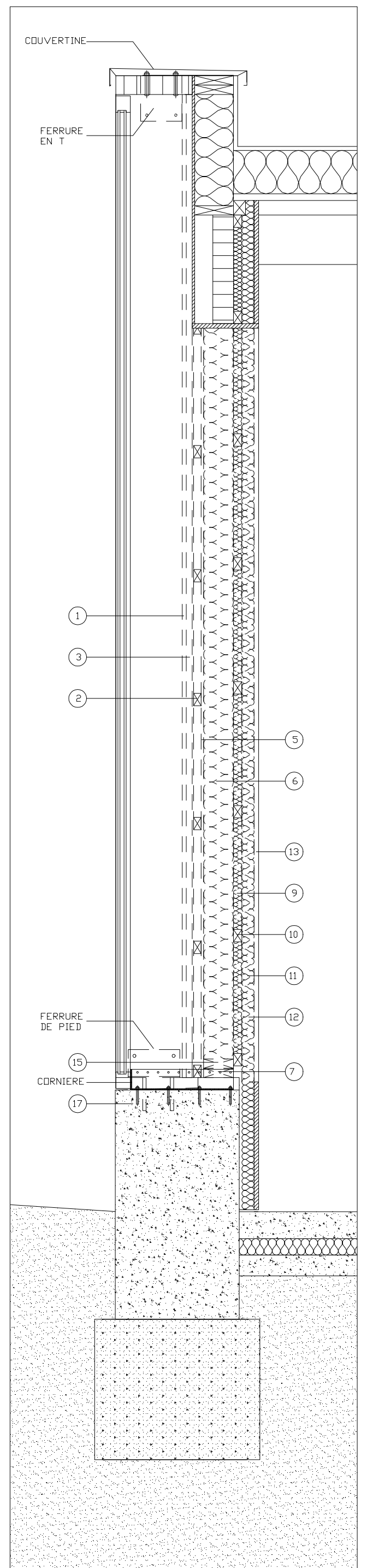
COUPE D 1_20
