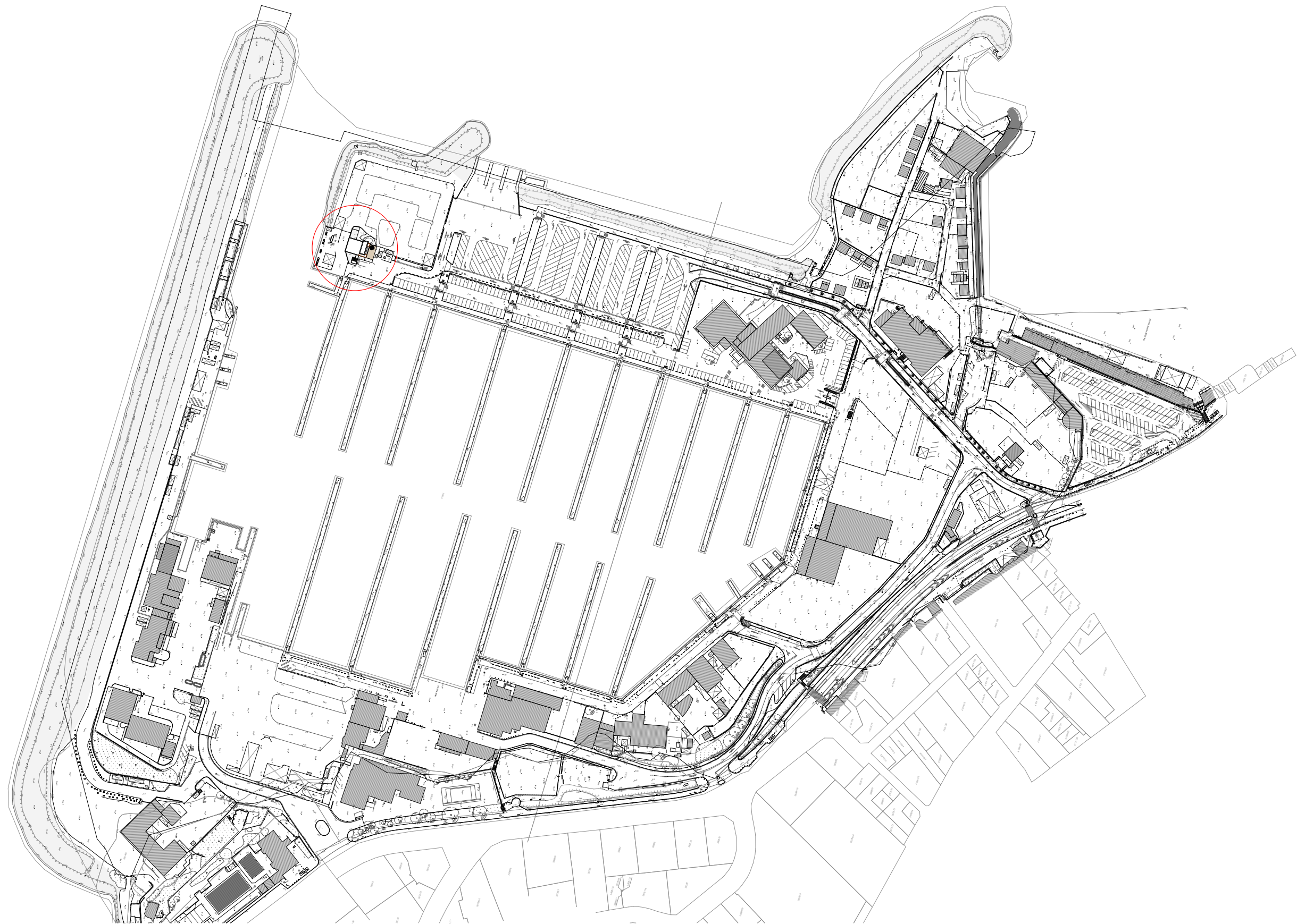
Projet - Plan masse du port de la Pointe Rouge 1:2500
