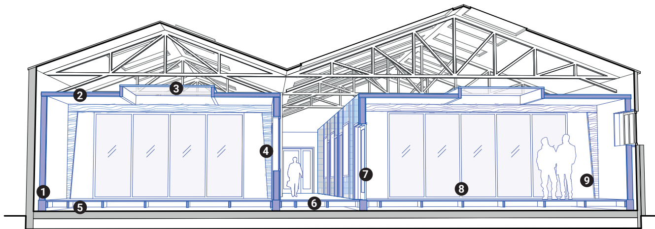
Coupe perspective sur les boîtes
