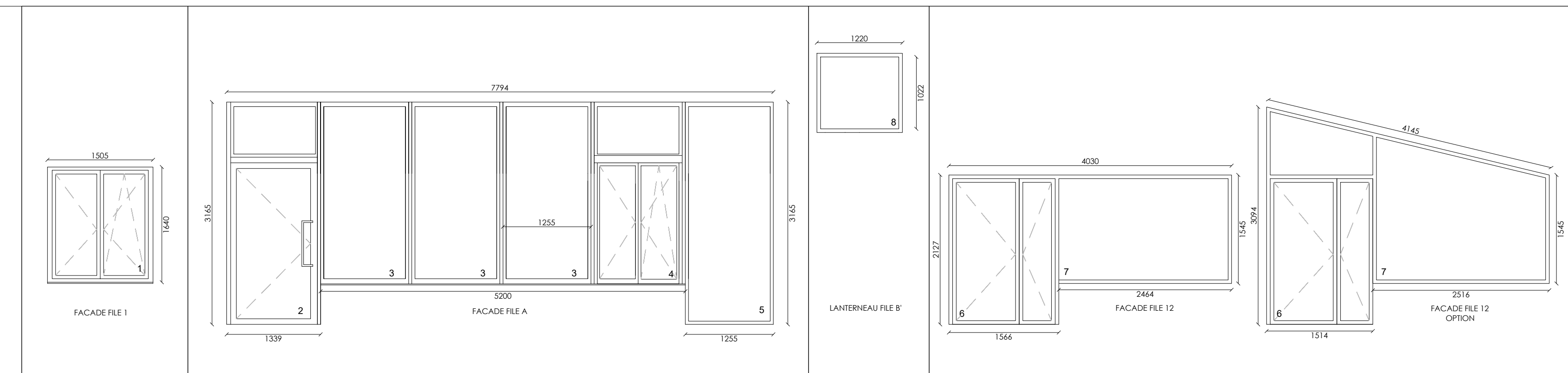
LOTS/ NOMENCLATURE MENUISERIE EXT: Toutes les menuiseries sont en ALU recyclé teinte au choix de l'architecte 1:50
