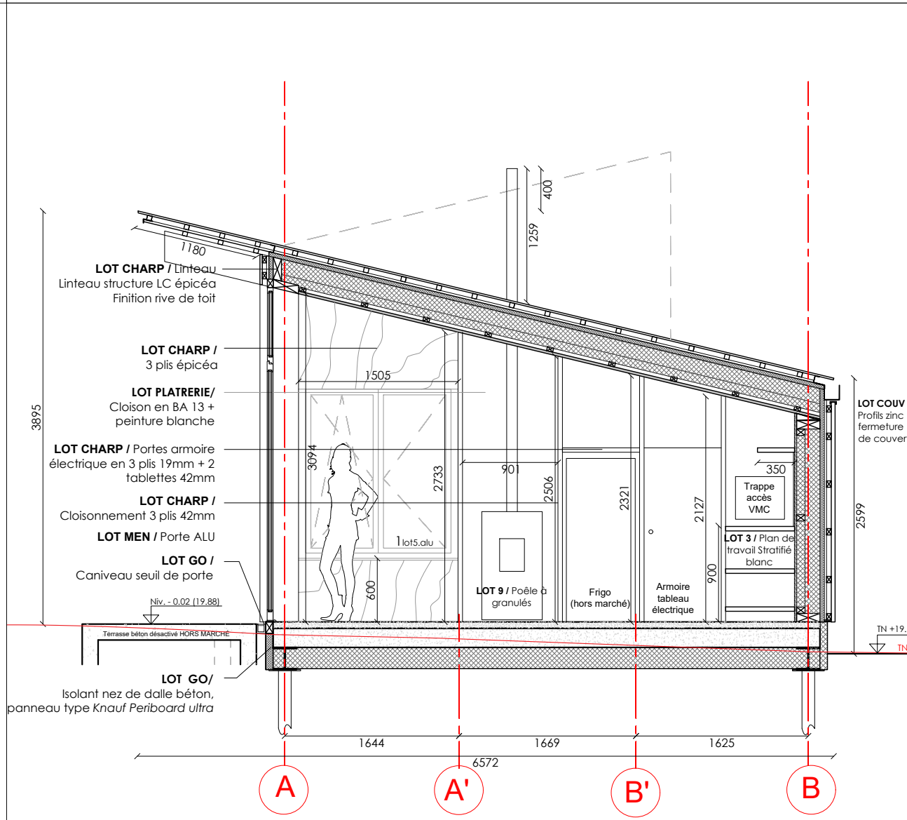
COUPE TRANSVERSALE 4 1:50
