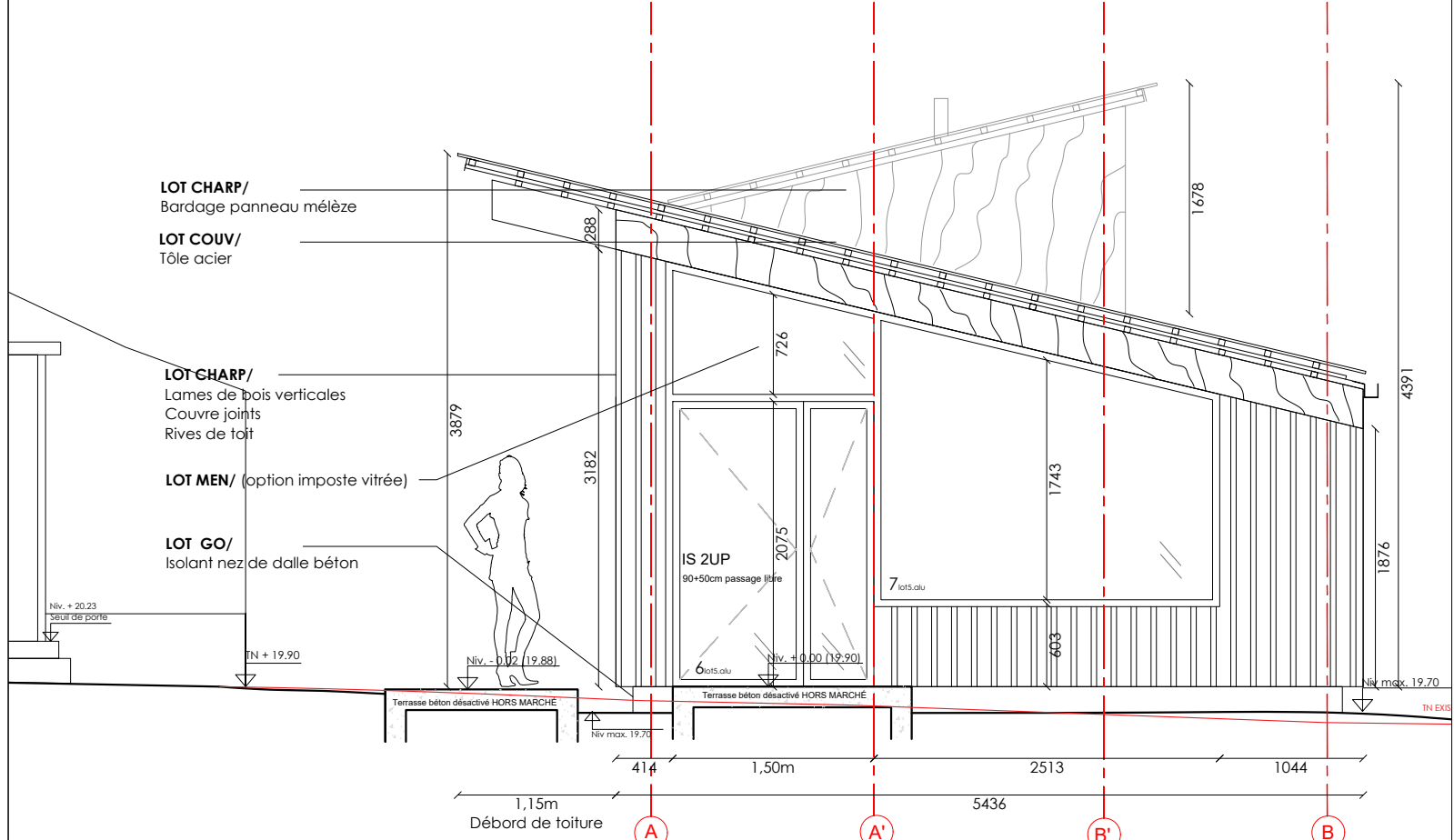
ELEVATION SUD - EST | FILE 12 (option imposte vitrée) 1:50
