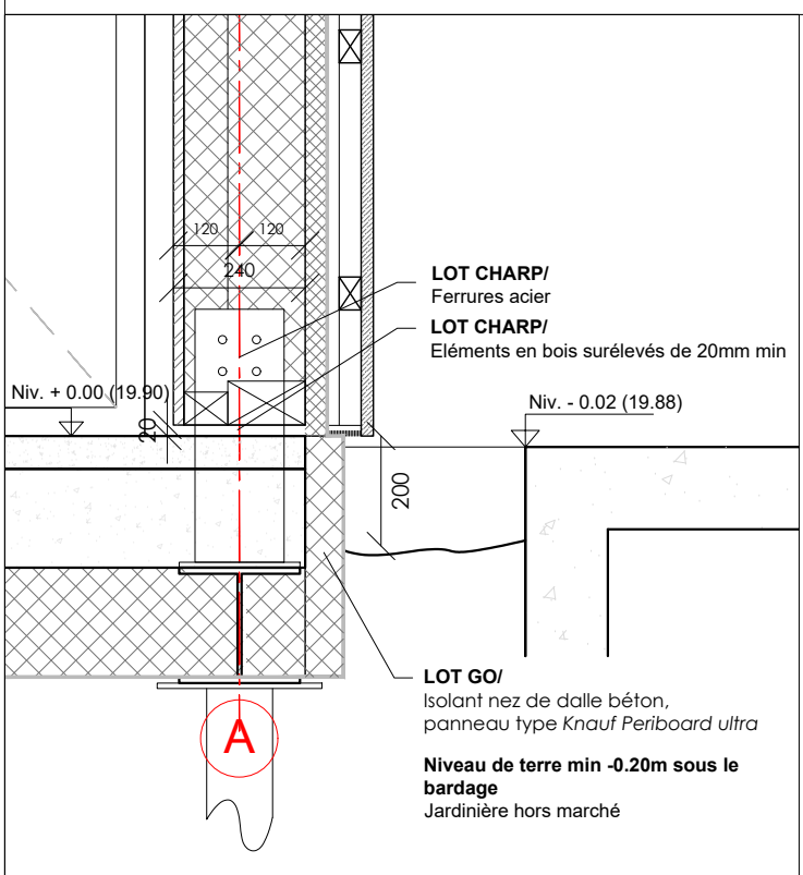
DETAIL PIED DE POTEAU 1:15
