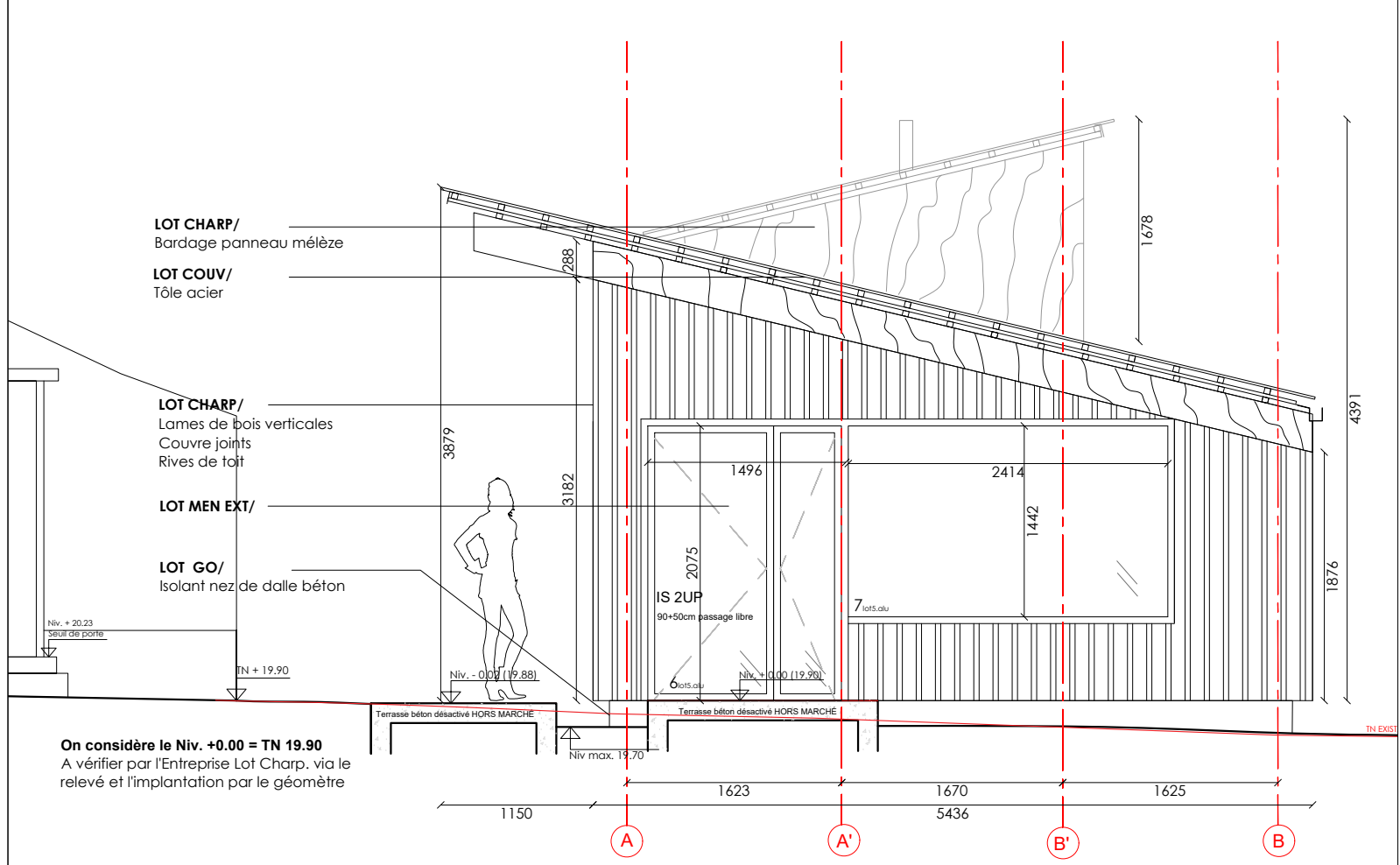
ELEVATION SUD - EST | FILE 12 1:50
