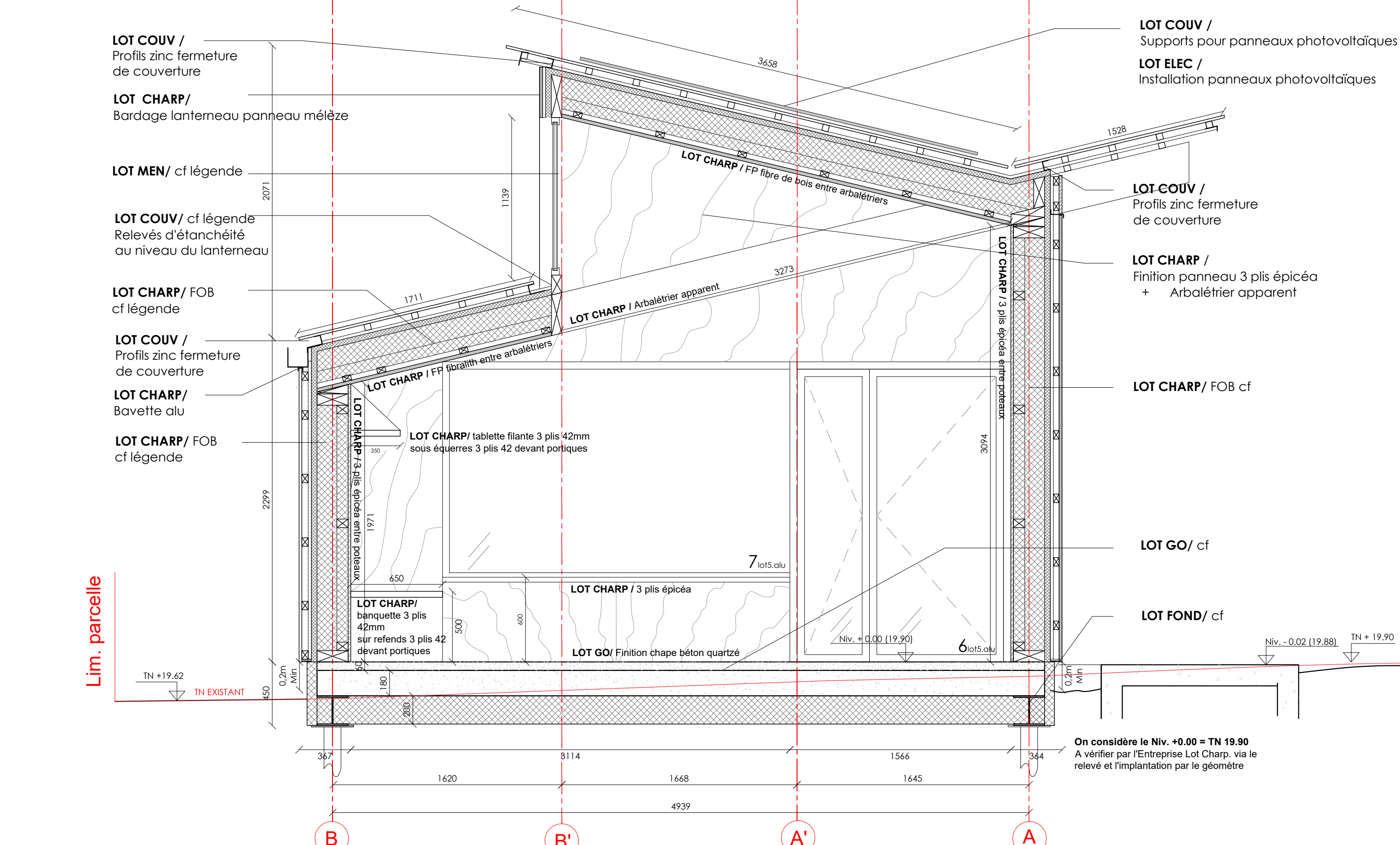
COUPE TRANSVERSALE FILE 5 1:25
