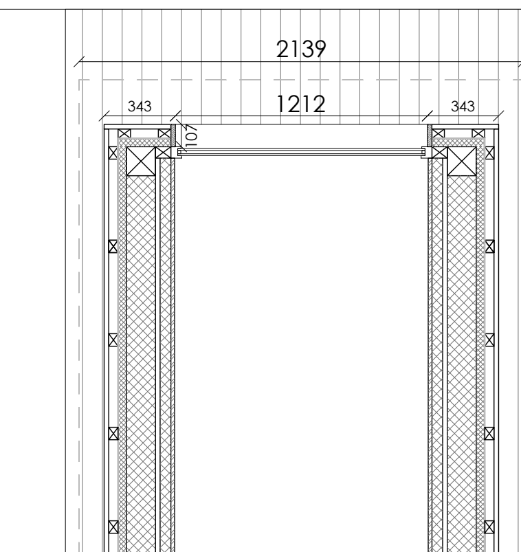
PLAN CHASSIS LANTERNEAU 1:25
