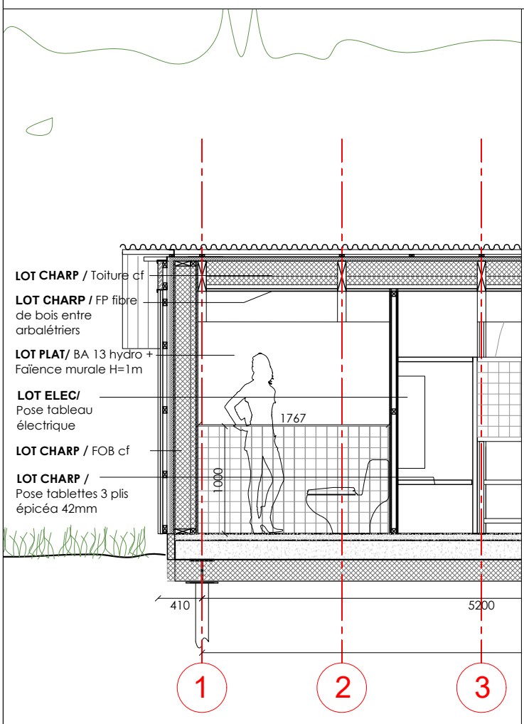
COUPE LONGITUDINALE C 1:50
