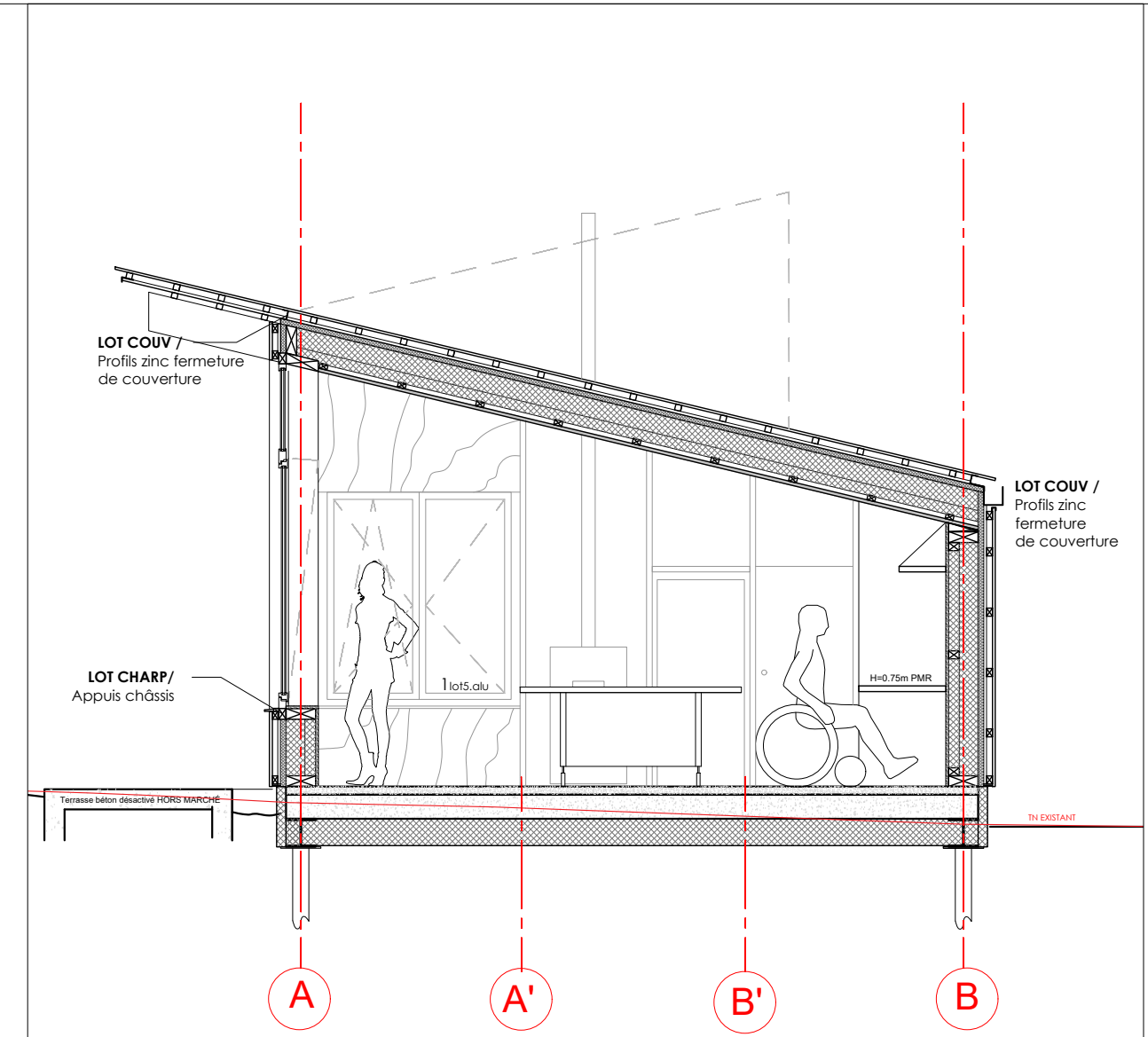
COUPE TRANSVERSALE 3 1:50
