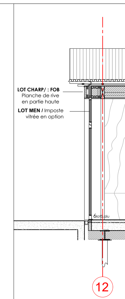
OPTION IMPOSTE VITRÉE 1:50
