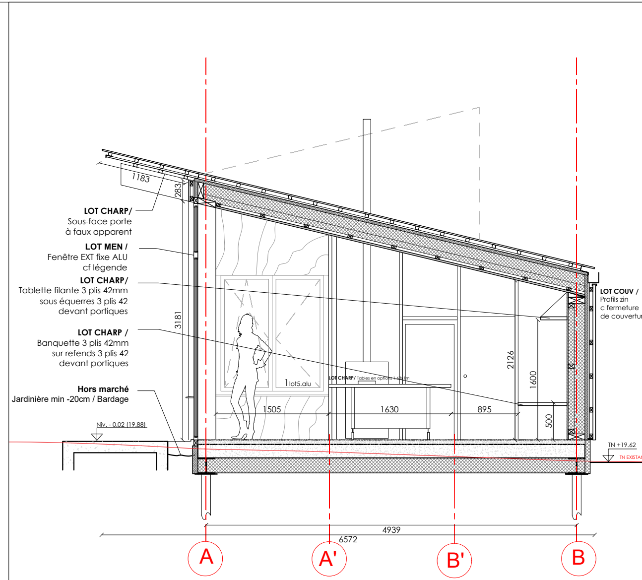
COUPE TRANSVERSALE 2 1:50
