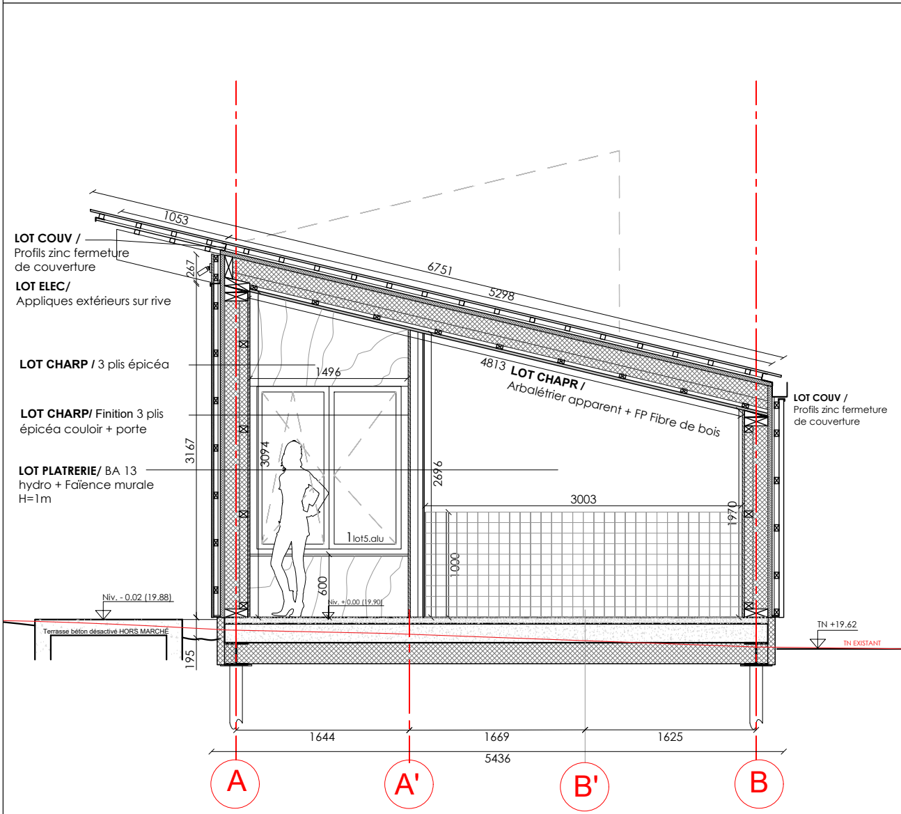
COUPE TRANSVERSALE 1 1:50
