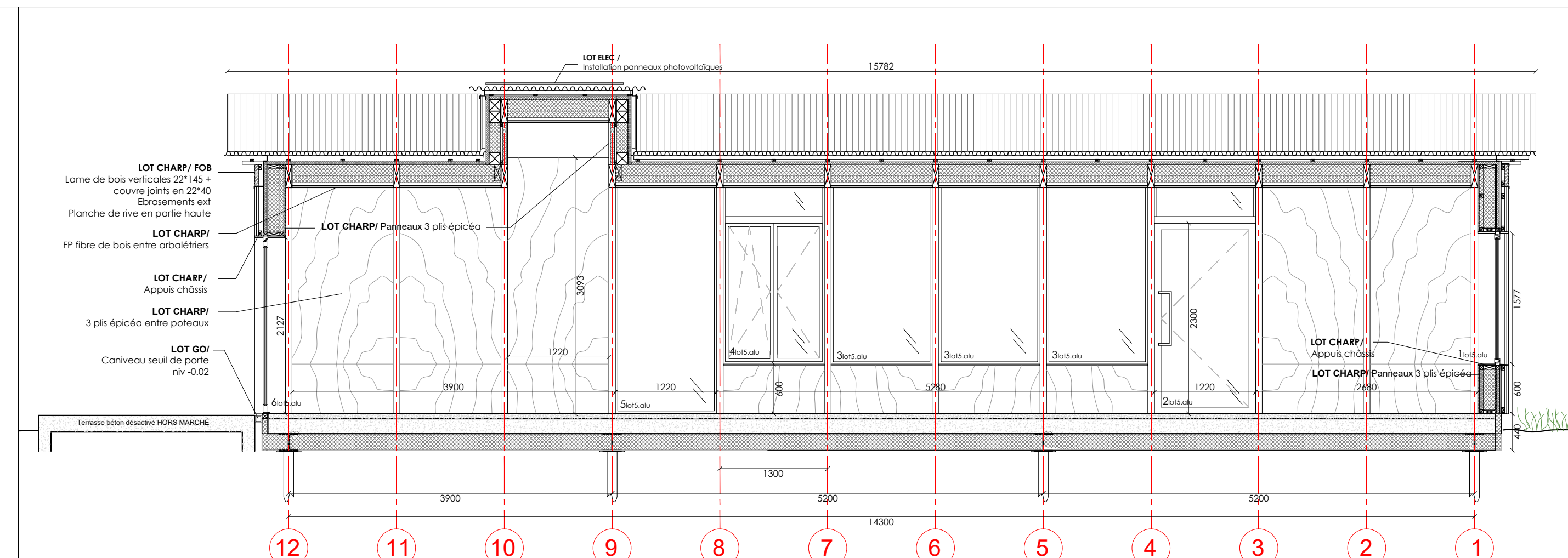
COUPE LONGITUDINALE A 1:50
