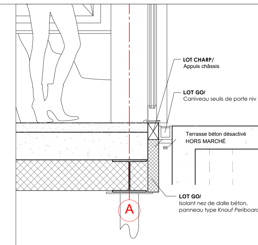
DETAIL PIED DE MENUISERIE EXT 1:15
