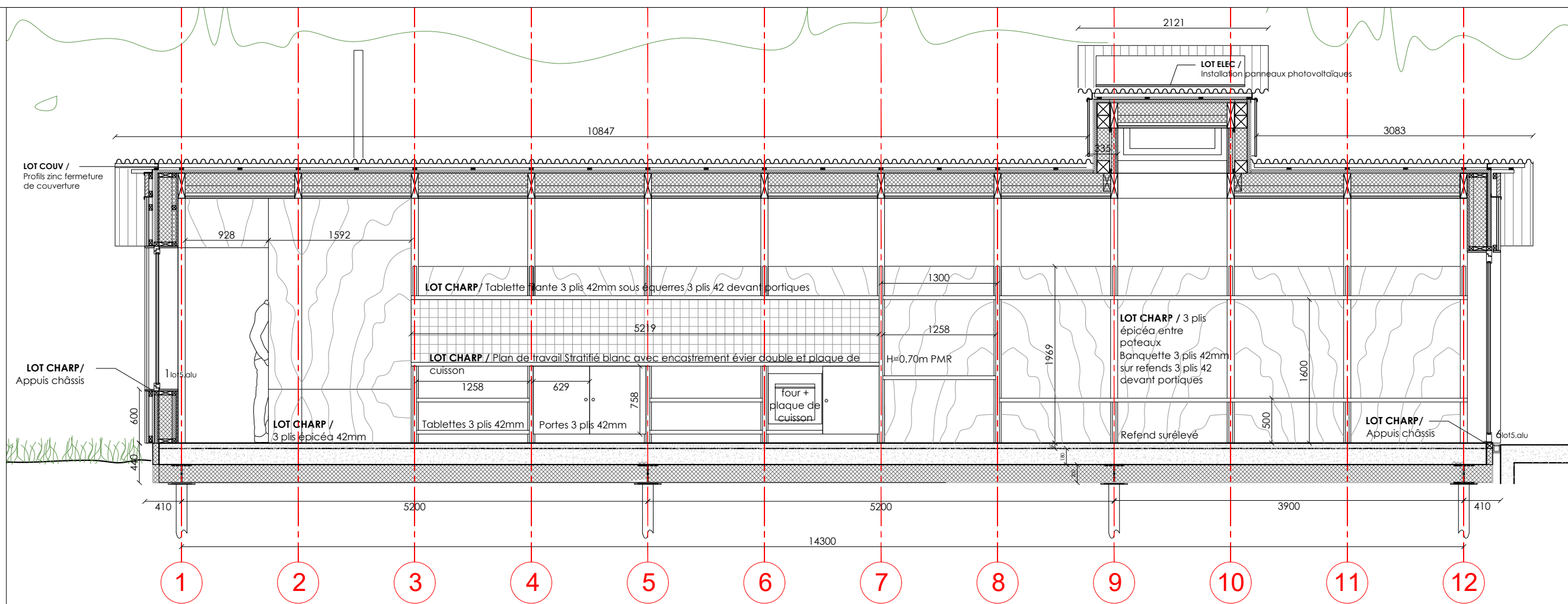
COUPE LONGITUDINALE B 1:50
