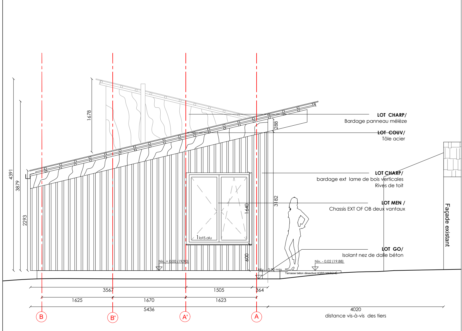
ELEVATION NORD - OUEST | FILE 1 1:50
