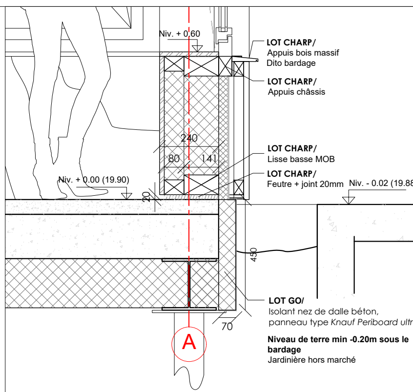
DETAIL PIED DE FOB 1:15
