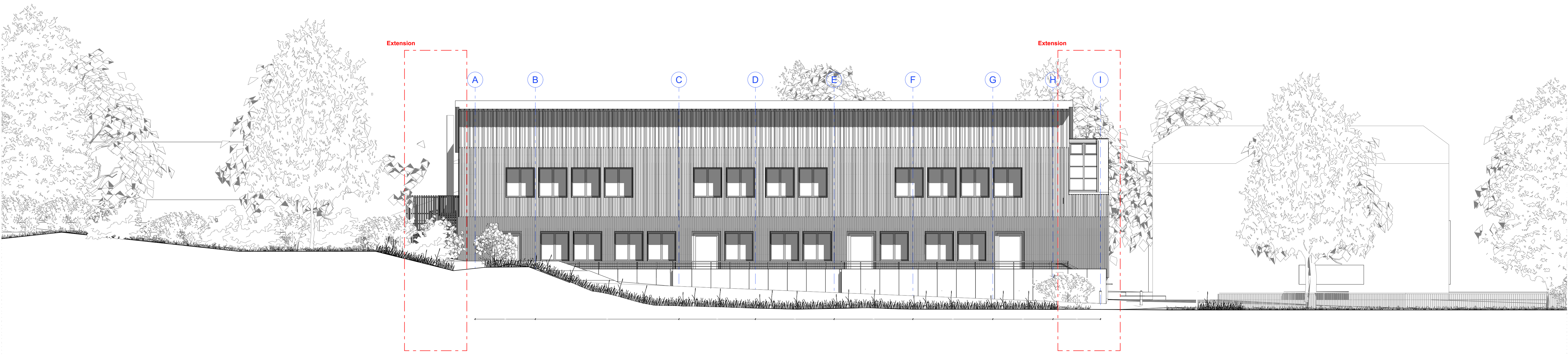
Façade Sud - Coupe paysagère - 1/100e
