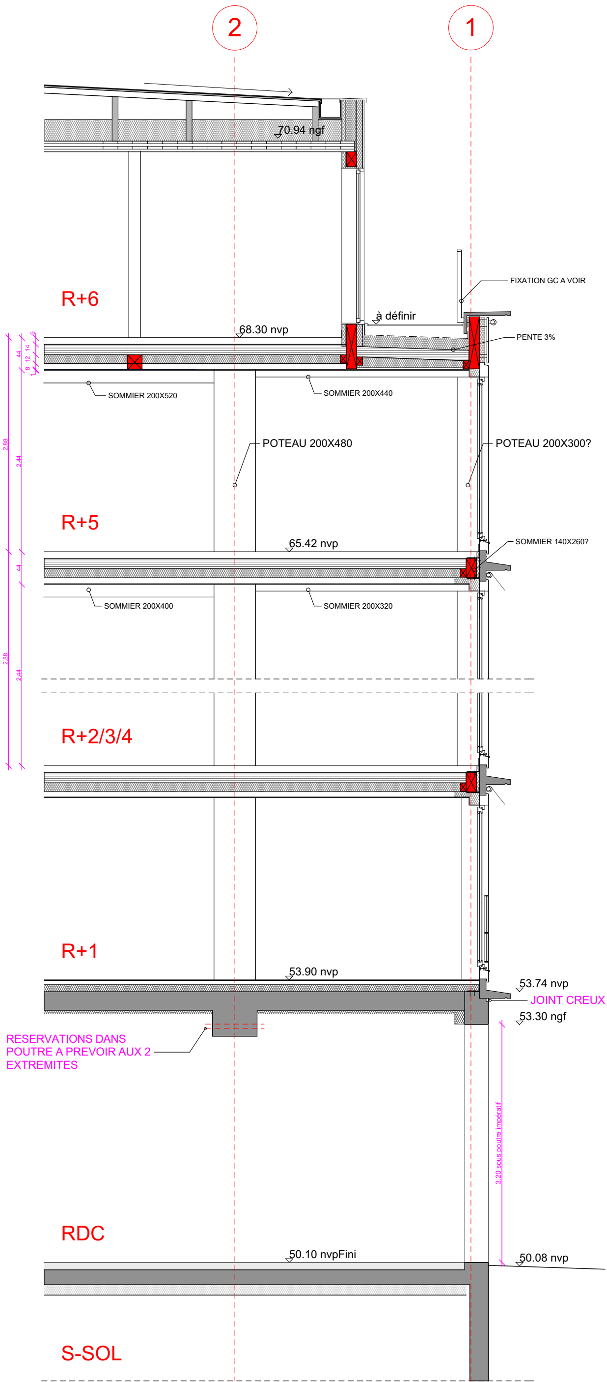
COUPE PHASE CHANTIER Modification planchers suite intégration doctrine pompiers
