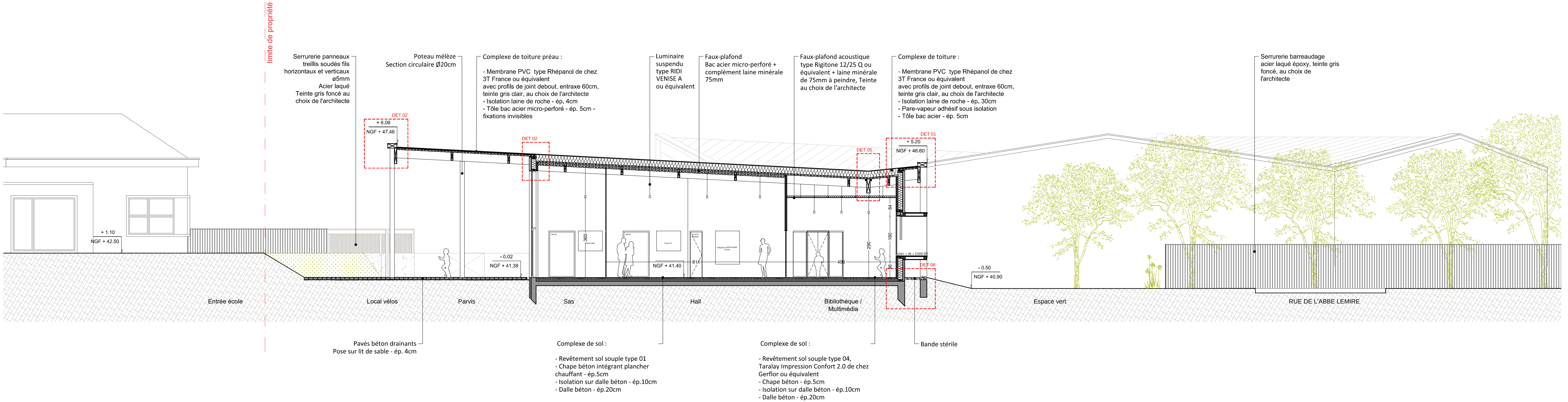
COUPE FF _ 1/100
