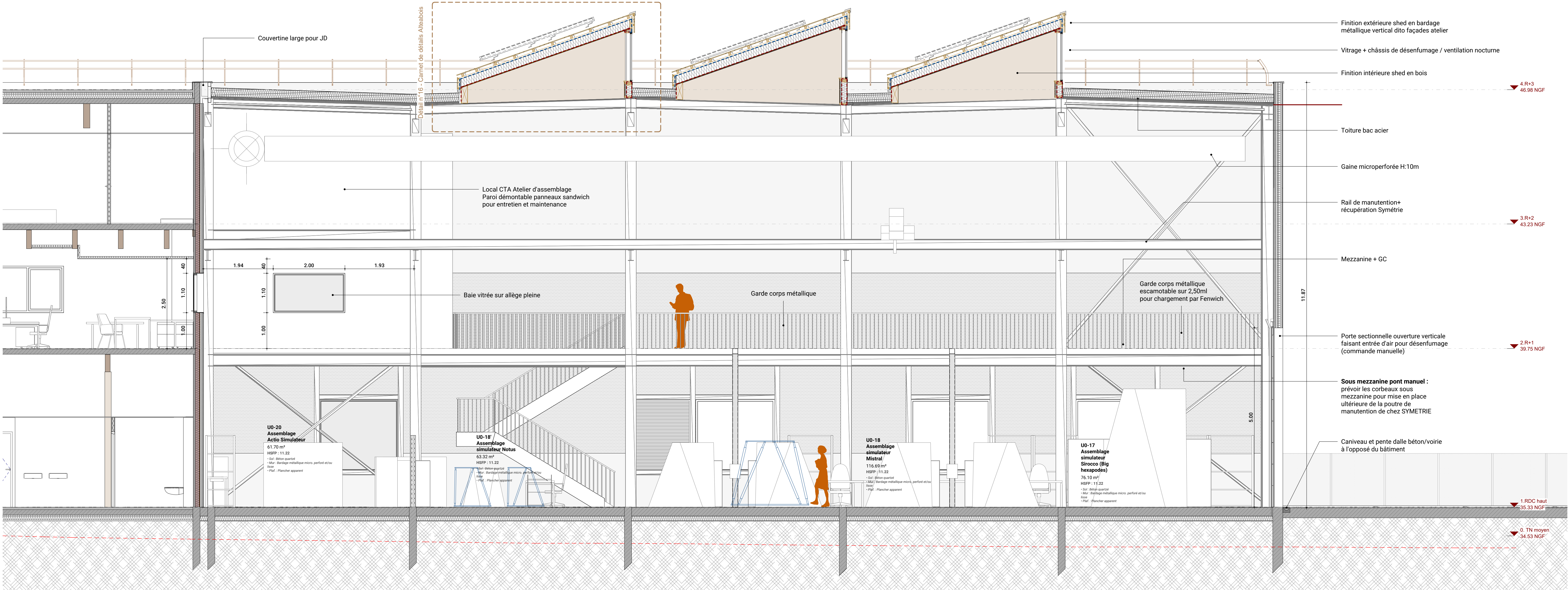
1 Coupe E' Longitudinal 50ème 1 : 50
