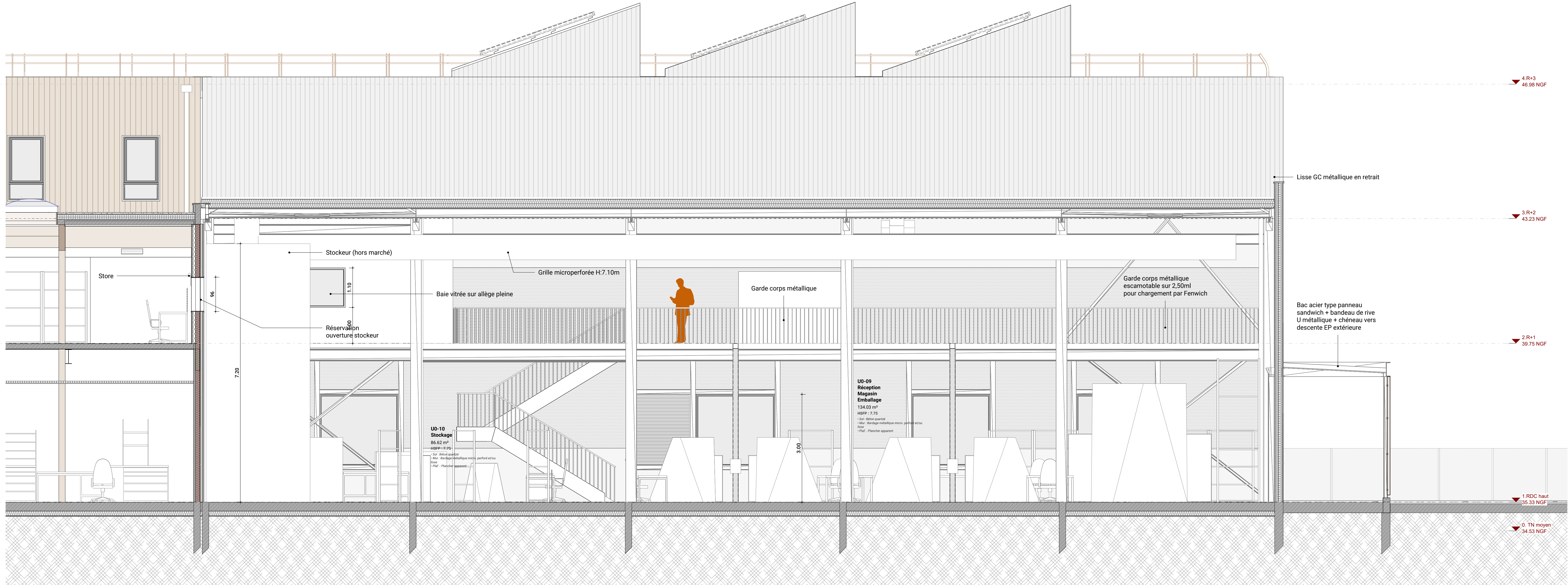
2 Coupe F' Longitudinal 50ème 1 : 50
