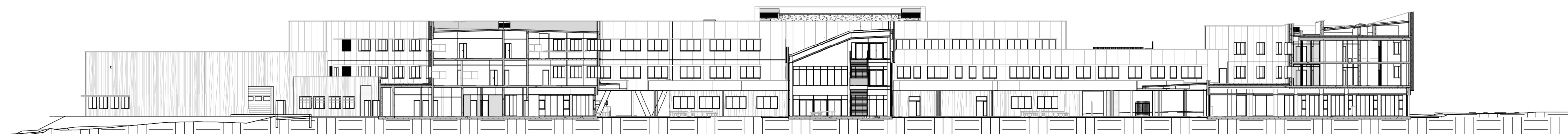
Coupe YY
