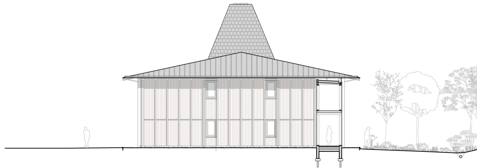
élévation nord
