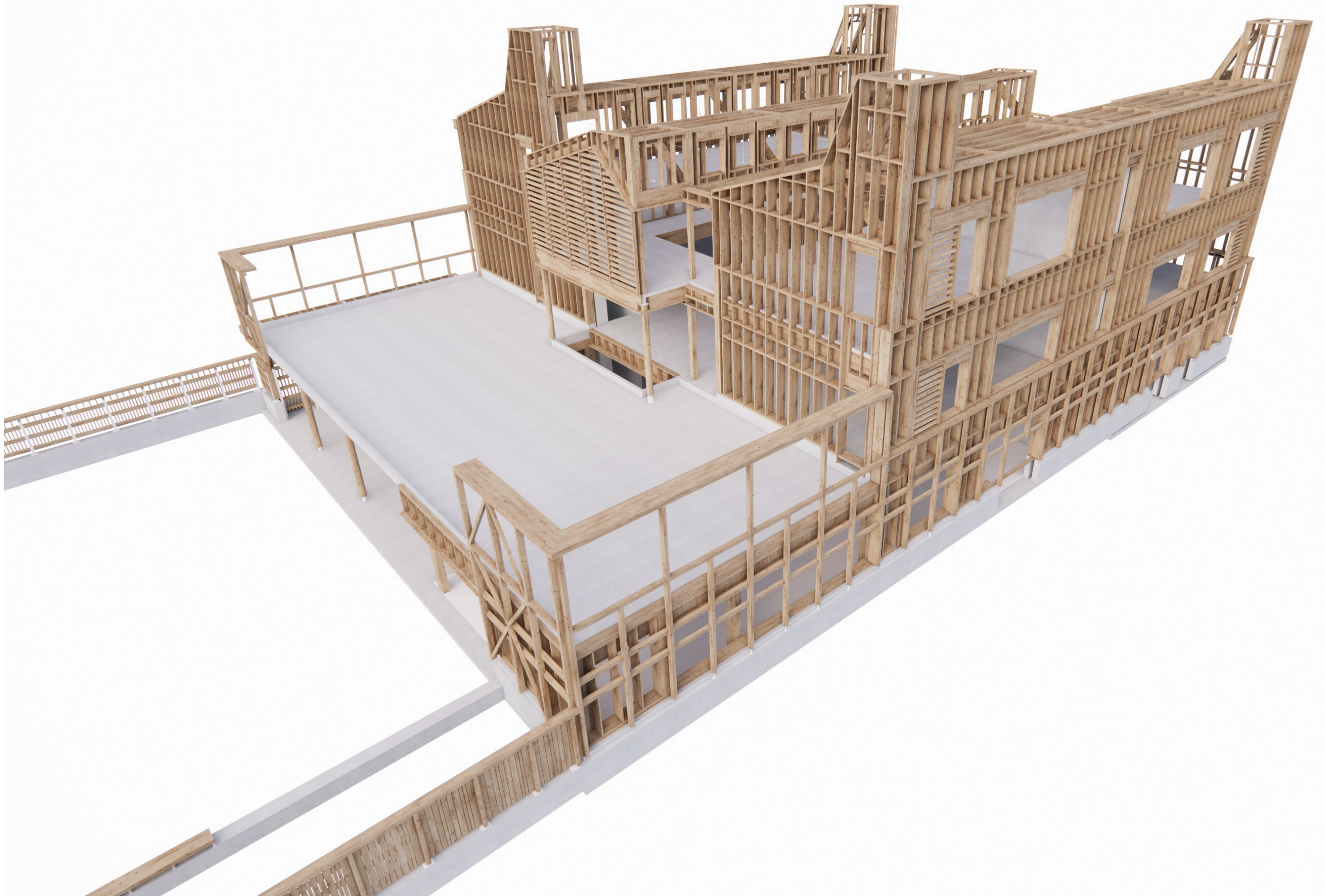
Perspective de l'ossature bois
