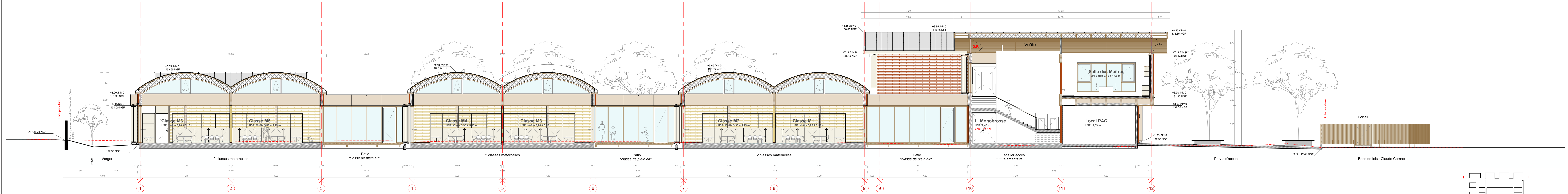
Coupe J - Salles de classe maternelle et cage d'escalier • 1 : 100
