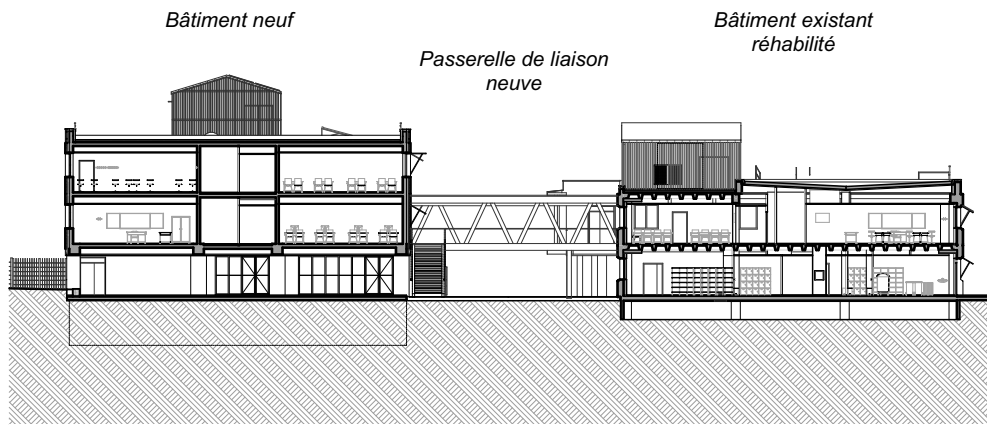
Coupe transversale
