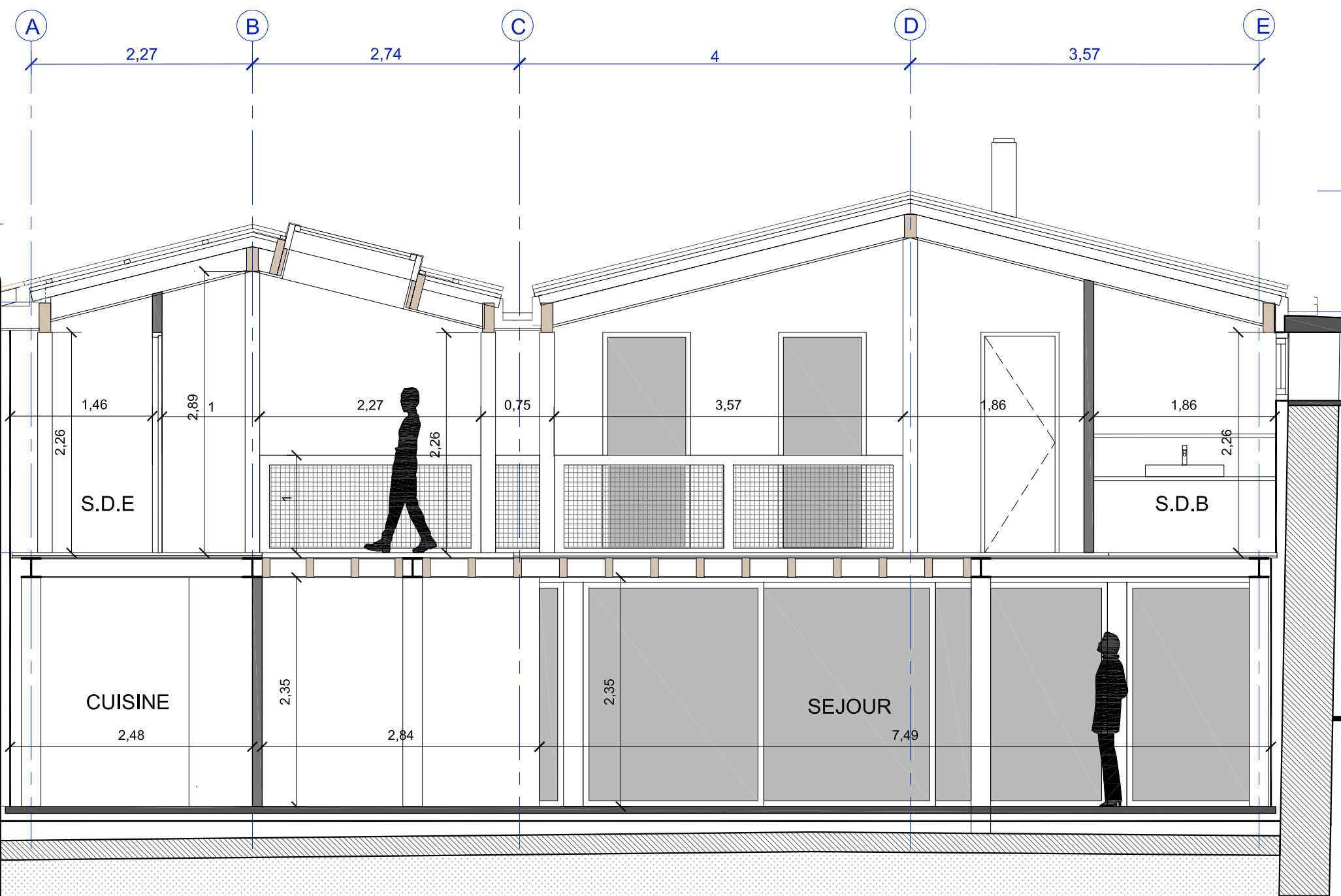
MAISON PK _ COUPE AA
