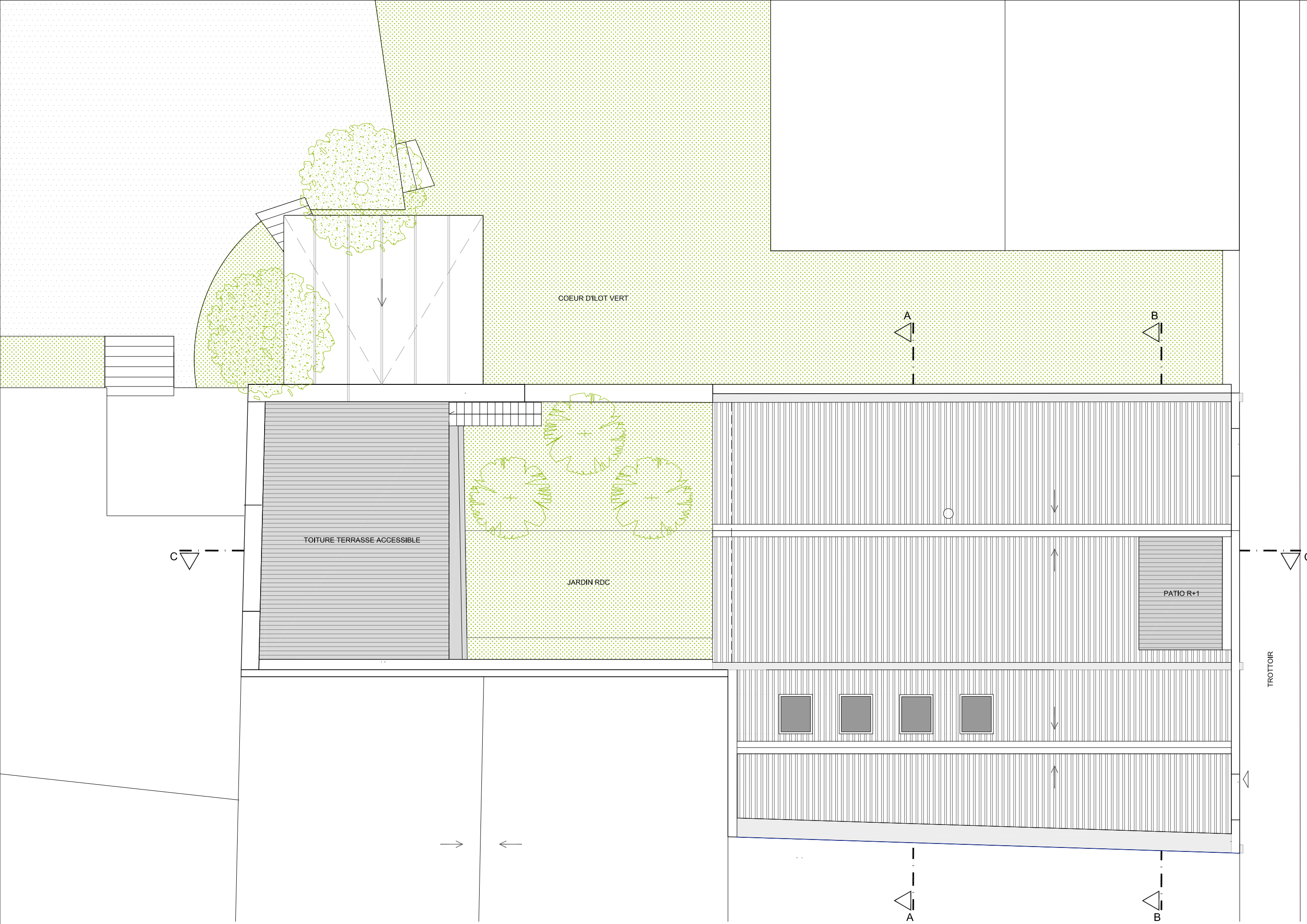
MAISON PK _ PLAN DE MASSE
