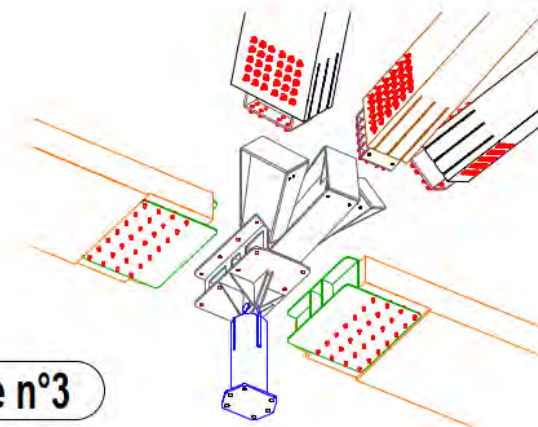
Vue dessous
