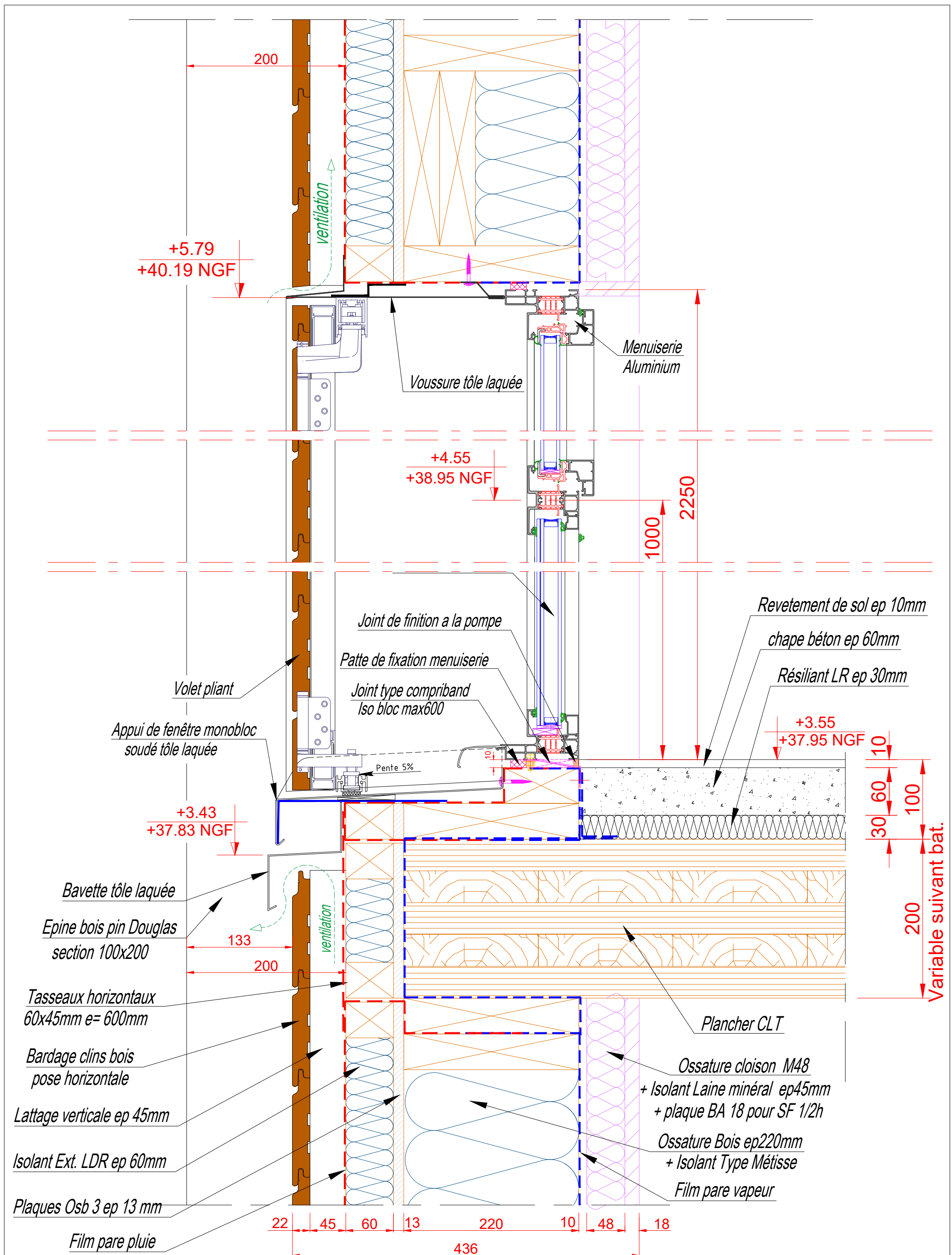
Coupe verticale sur fenêtre R+1 avec volet pliant
