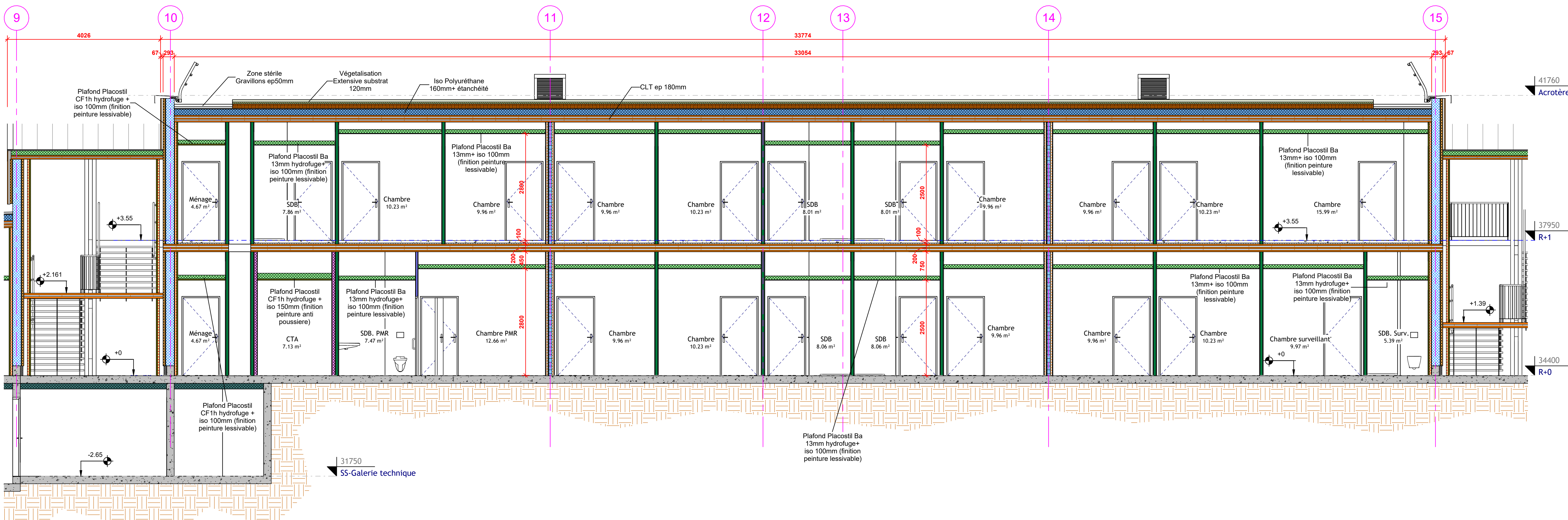
1 Coupe 1 Bat. 2.2 Ech : 1 : 50
