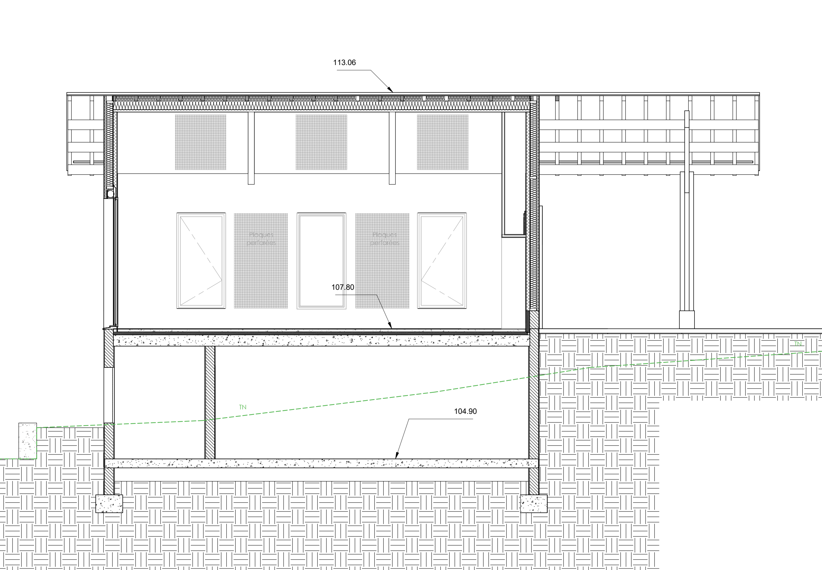
Coupe 03 - Echelle : 1/50
