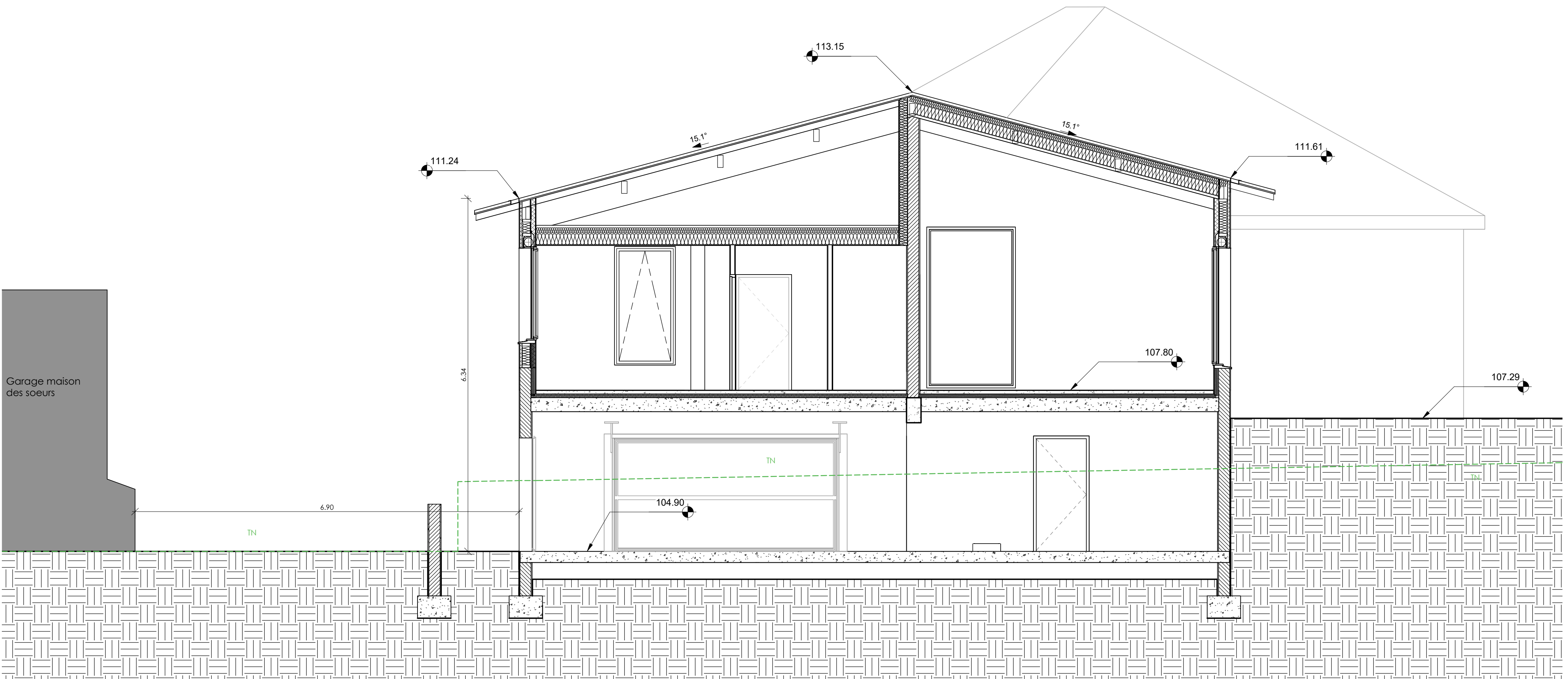
Coupe 02 - Echelle : 1/50
