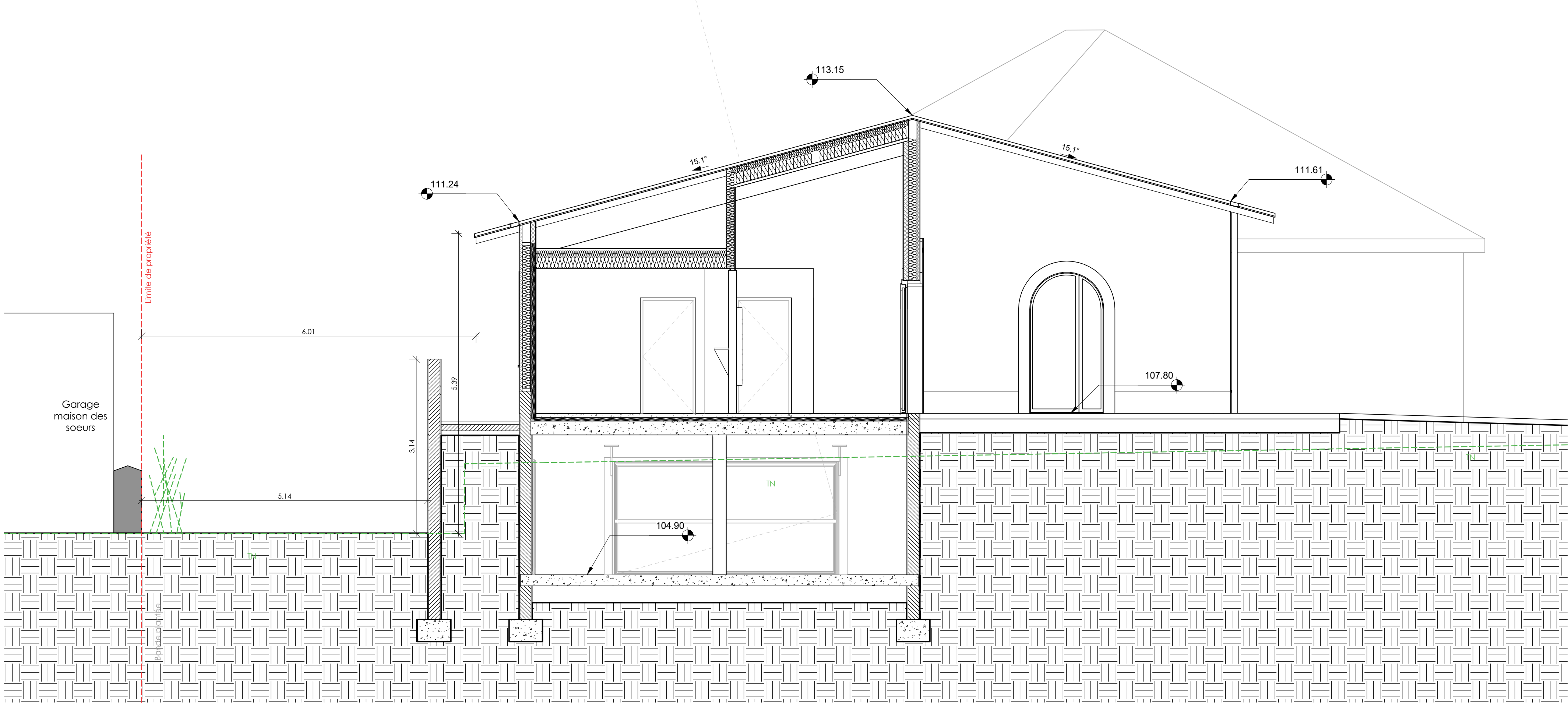
Coupe 01 - Echelle : 1/50
