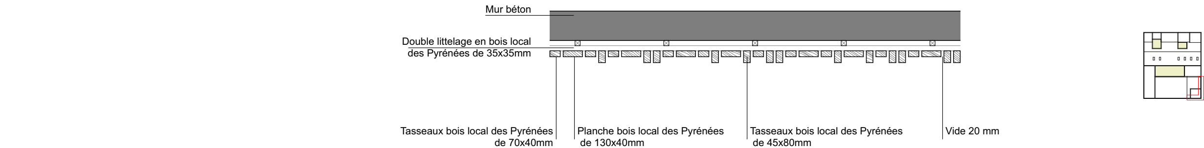
DÉTAILS EN PLAN BARDAGE BOIS SUR BÉTON_ Ech: 1/25 ème
