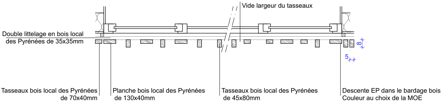
DÉTAILS EN PLAN CLAUSTRA BOIS_ Ech: 1/25 ème
