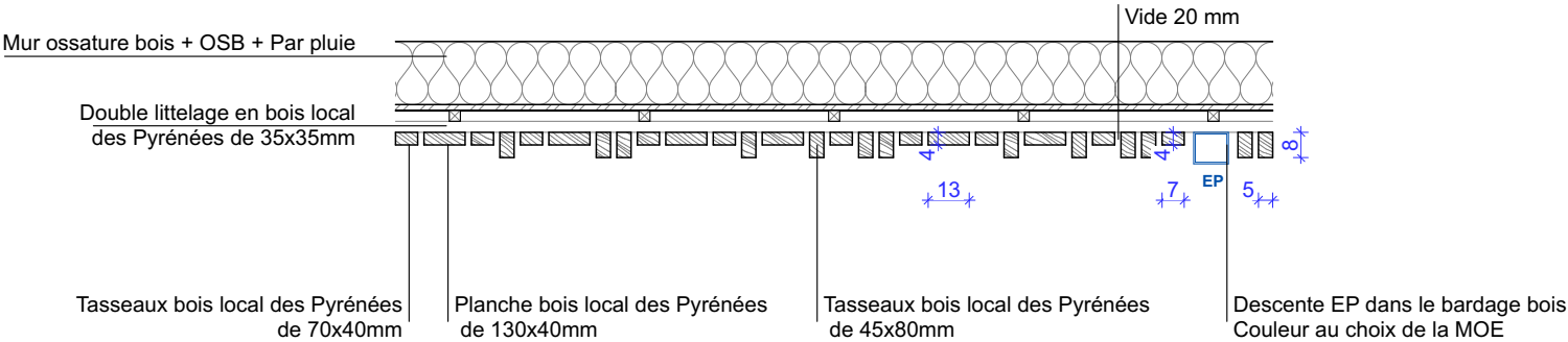
DÉTAILS EN PLAN BARDAGE BOIS SUR MOB_ Ech: 1/25 ème
