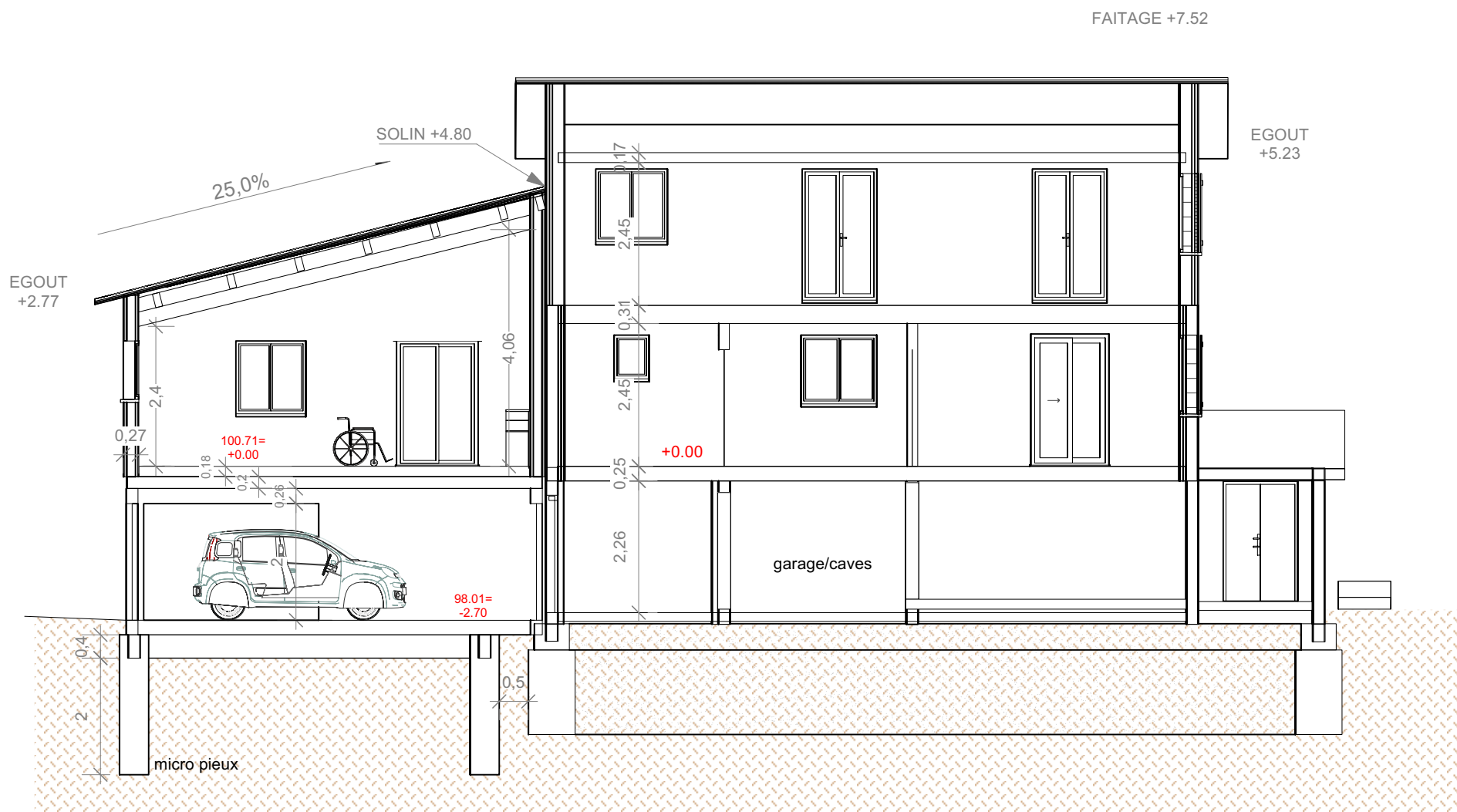
1 COUPE AA Échelle: 1:100
