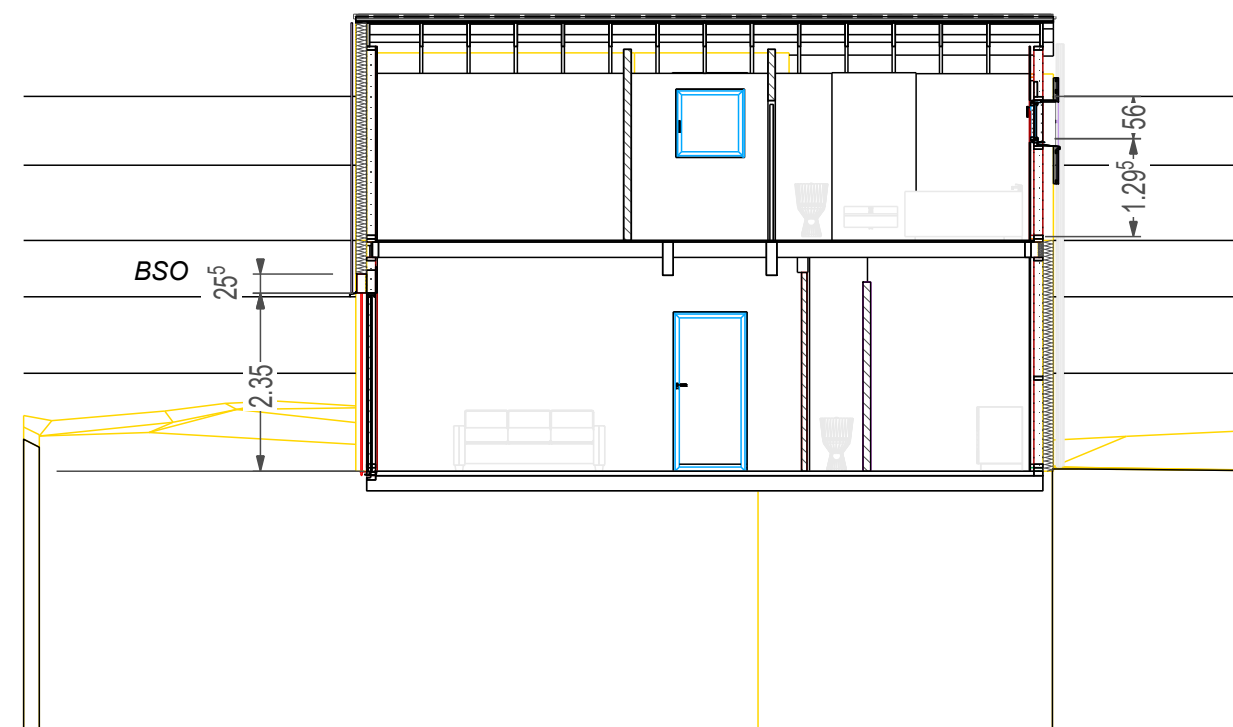
Coupe 1:100 B
