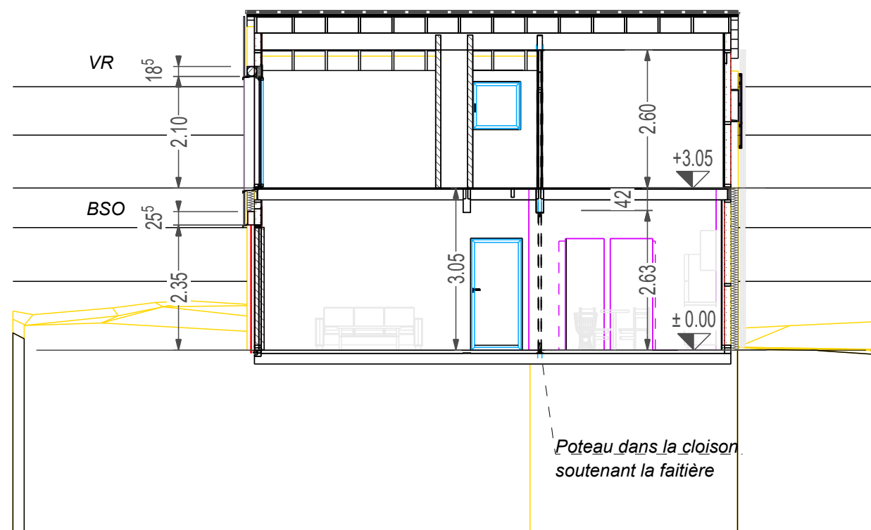
Coupe 1:100 A
