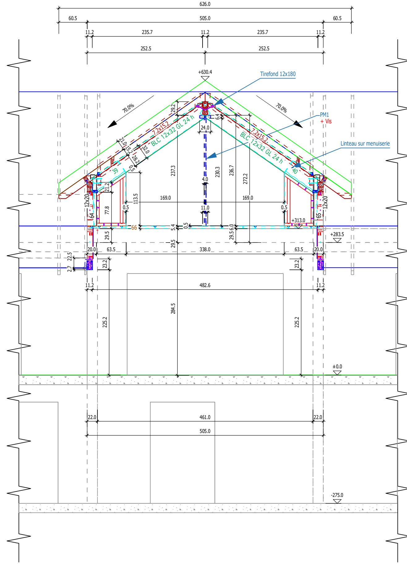
COUPE 2
