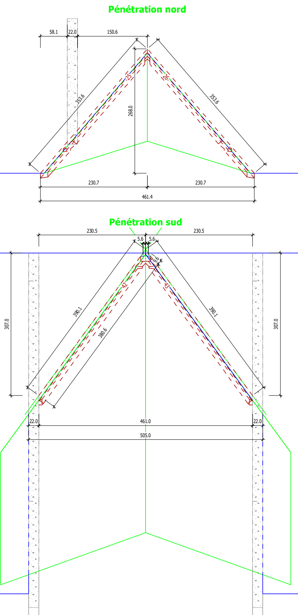
Cote au rampant pour découpe chevron existant
