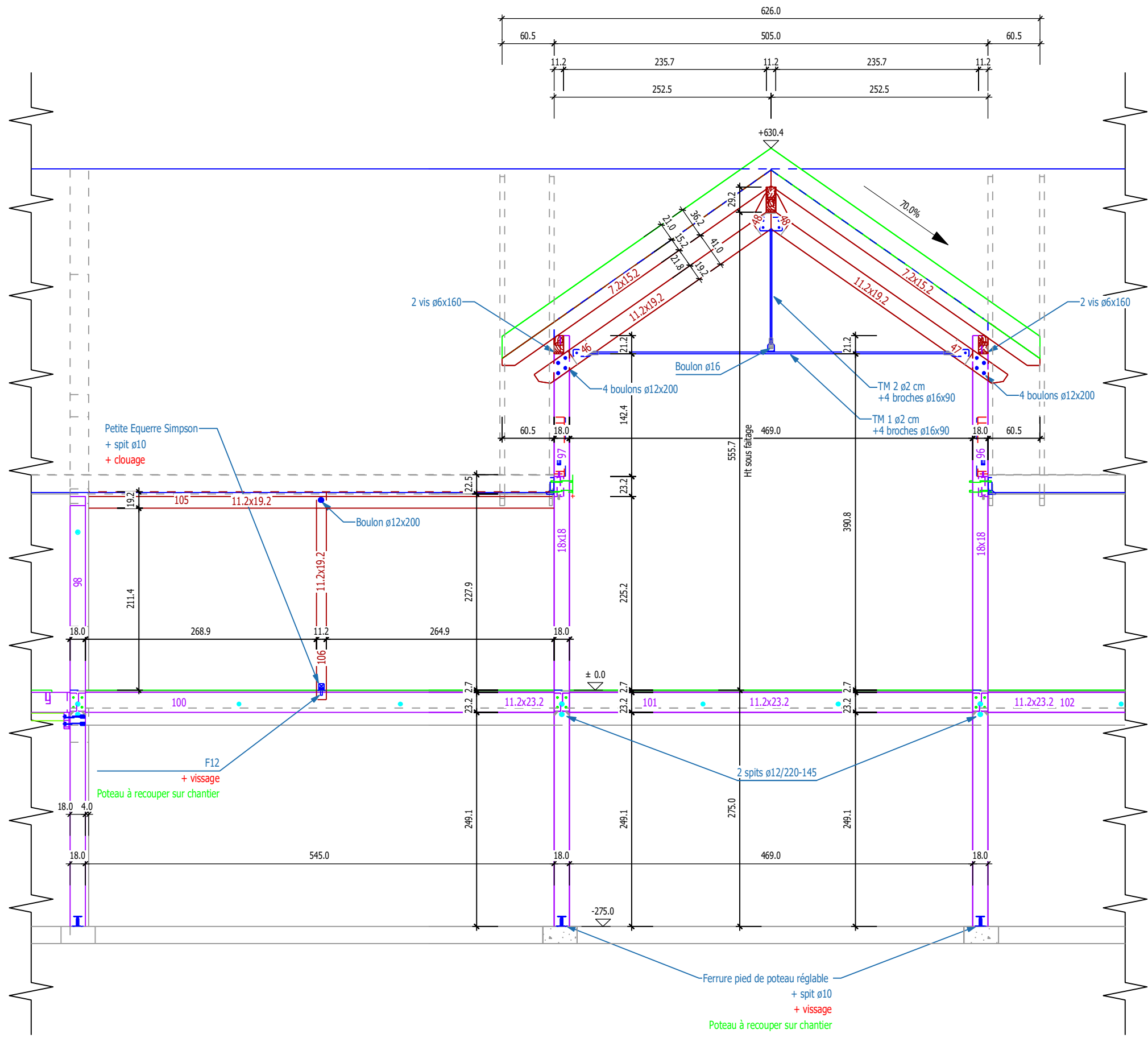
COUPE 1
