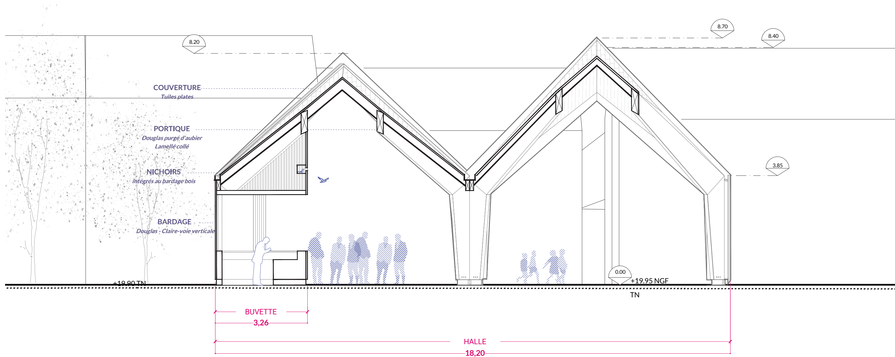
Coupe transversale
