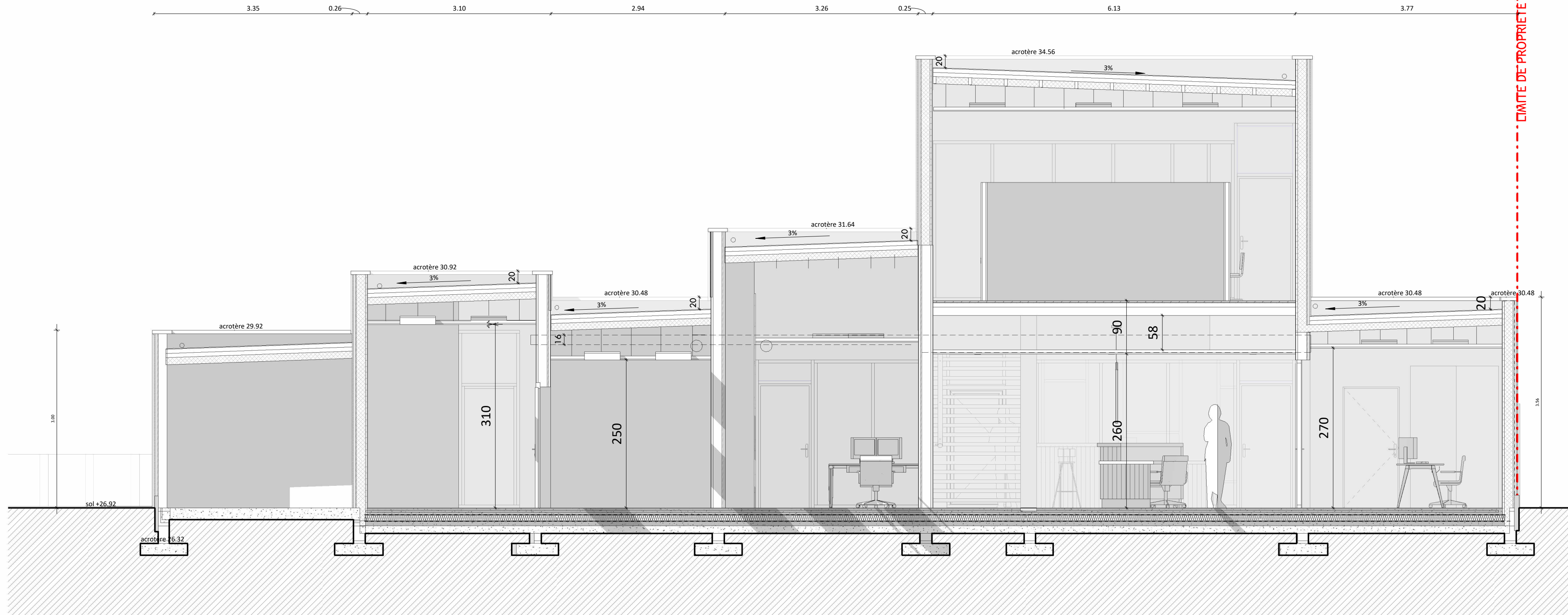
COUPE LONGITUDINALE - éch : 1 : 50
