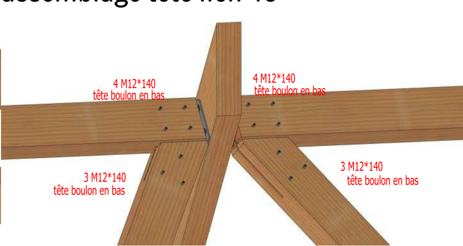
assemblage tête lien 40
