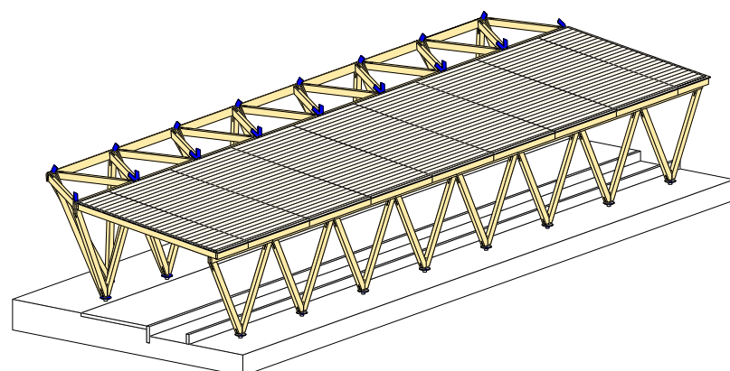
LEVAGE CAISSONS Structure stabilisée
