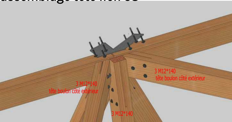
assemblage tête lien 58
