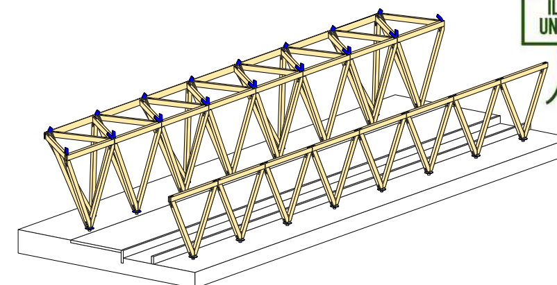
LEVAGE BIPODES Structure à étayer
