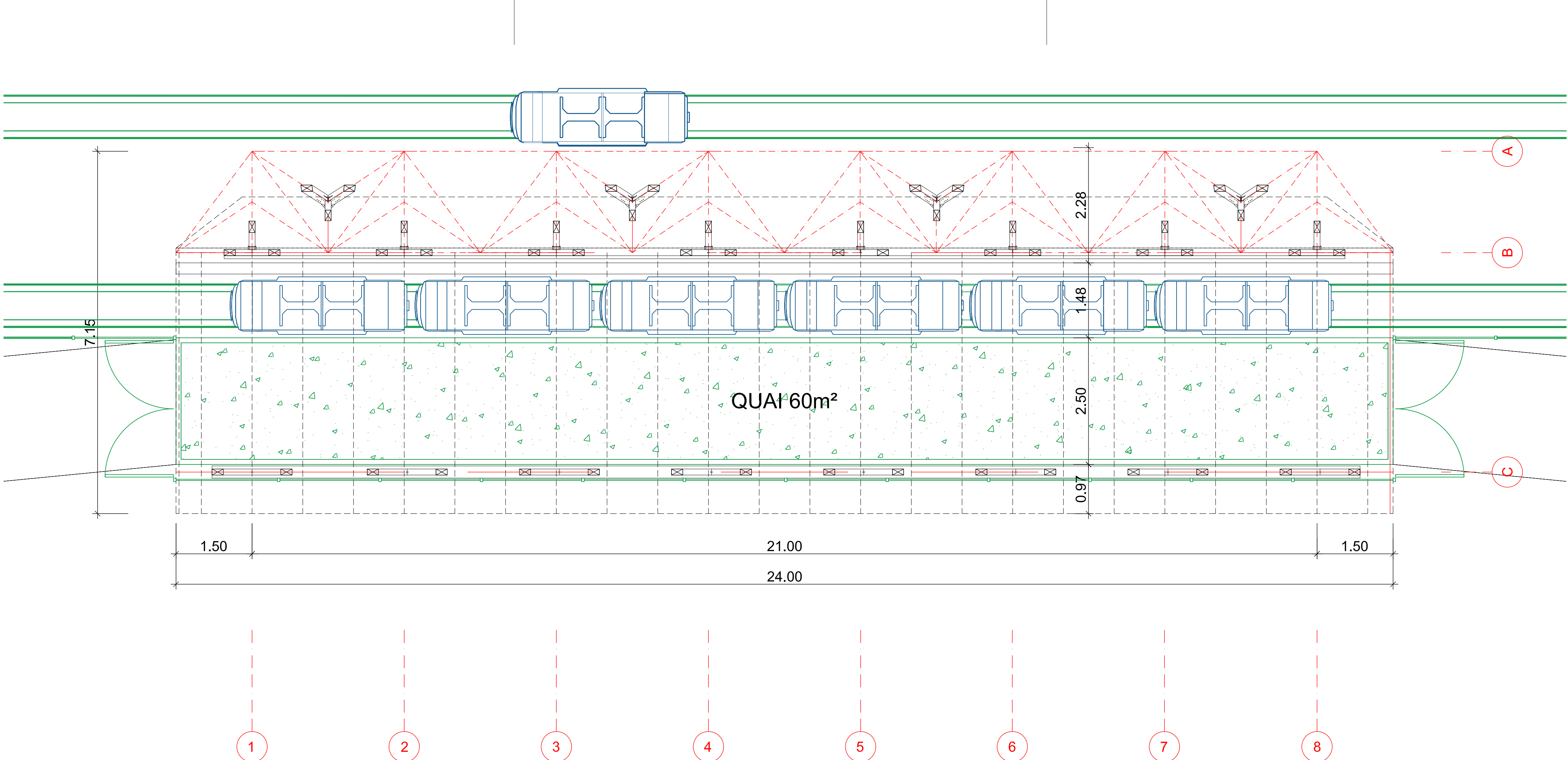
PLAN - ECH : 1/50
