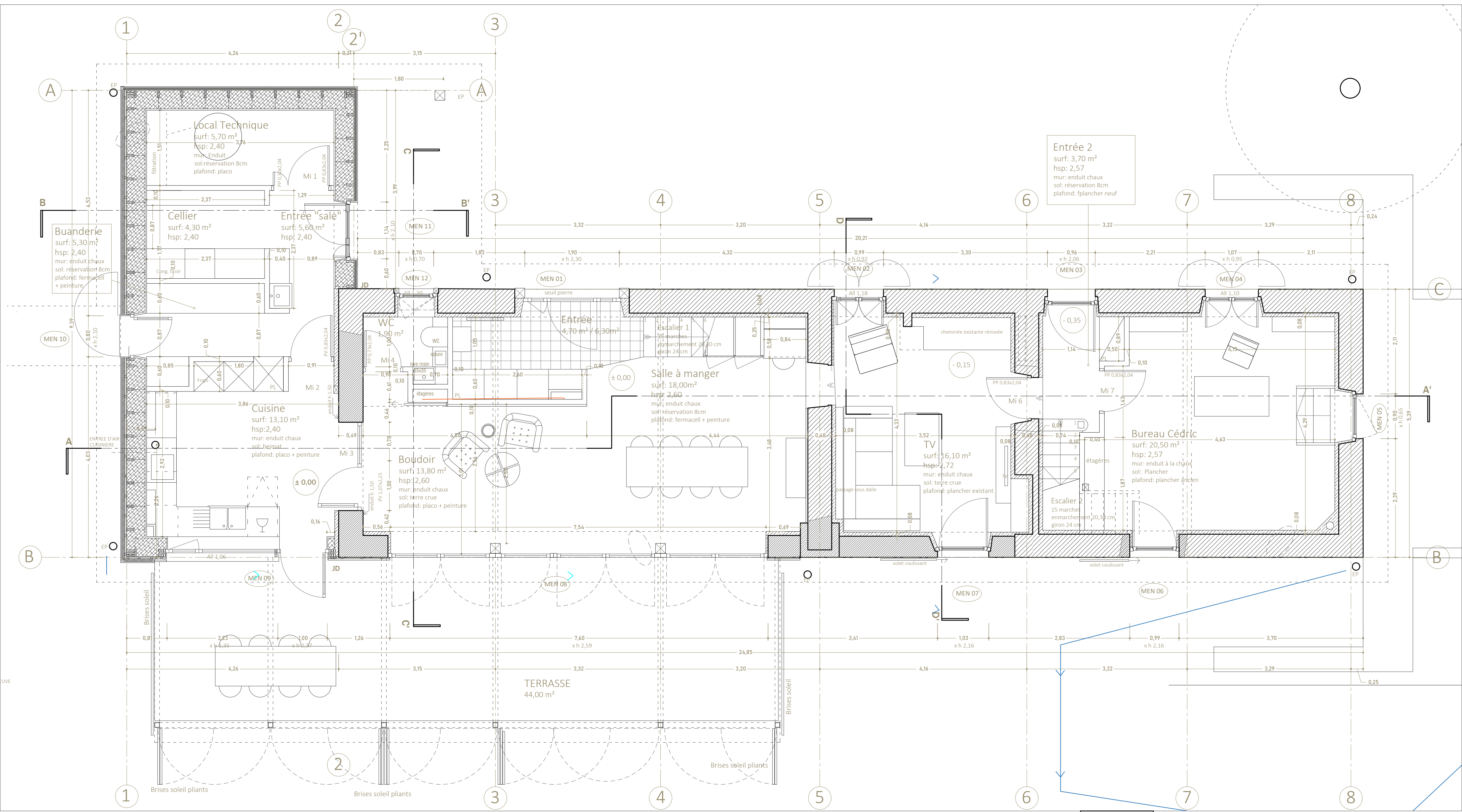
A 102 PLAN REZ-DE-CHAUSSEE échelle: 1/50
