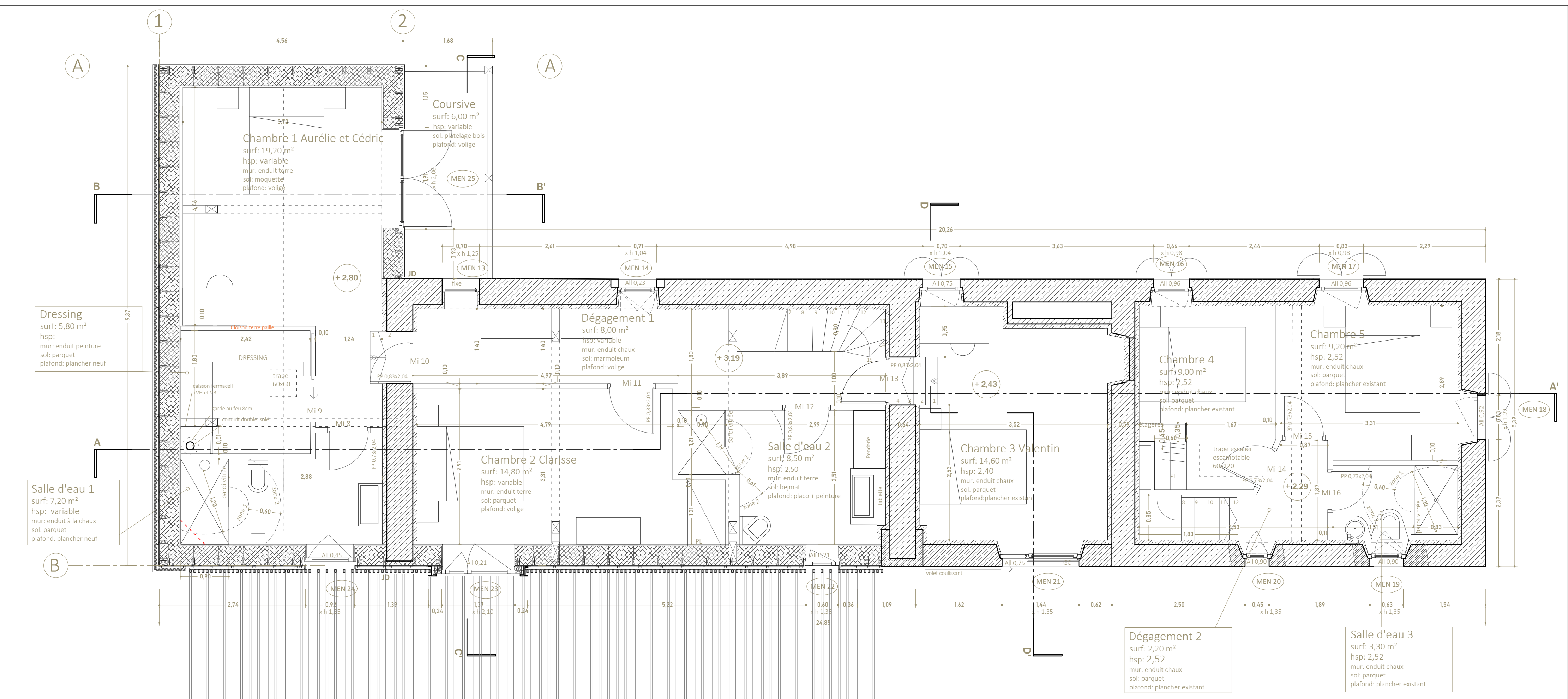
A 103 PLAN ETAGE échelle: 1/50
