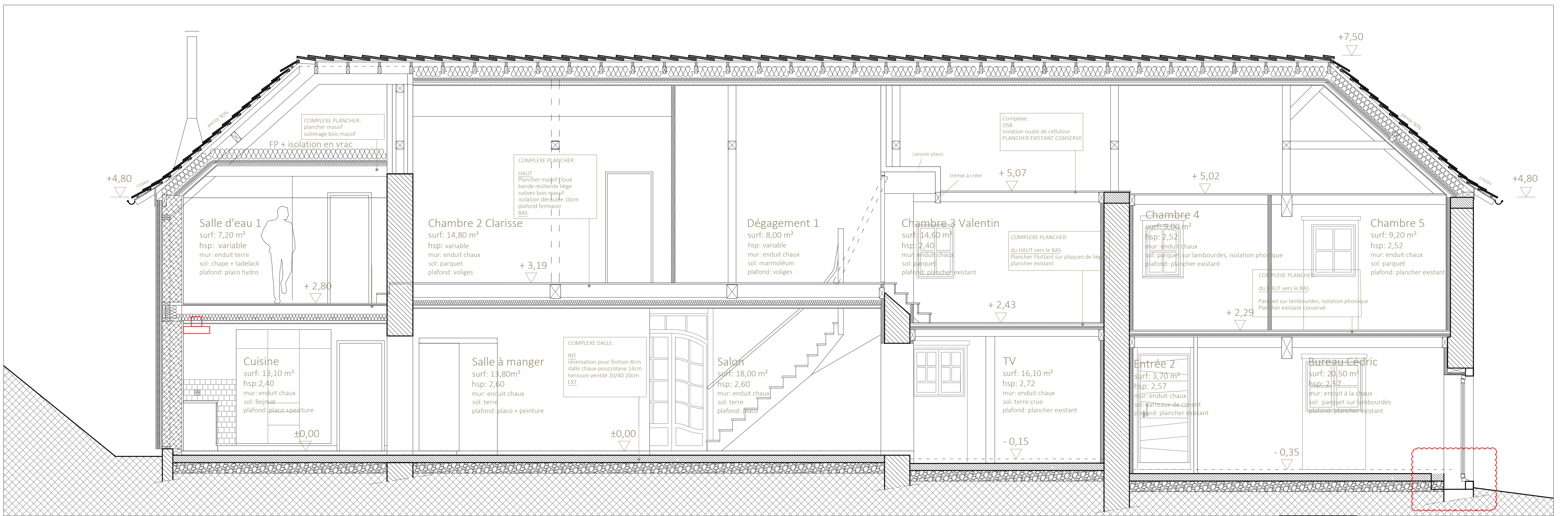
A 201 COUPE AA' échelle: 1/50
