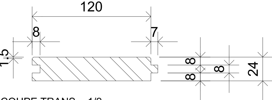
COUPE TRANS - 1/2
