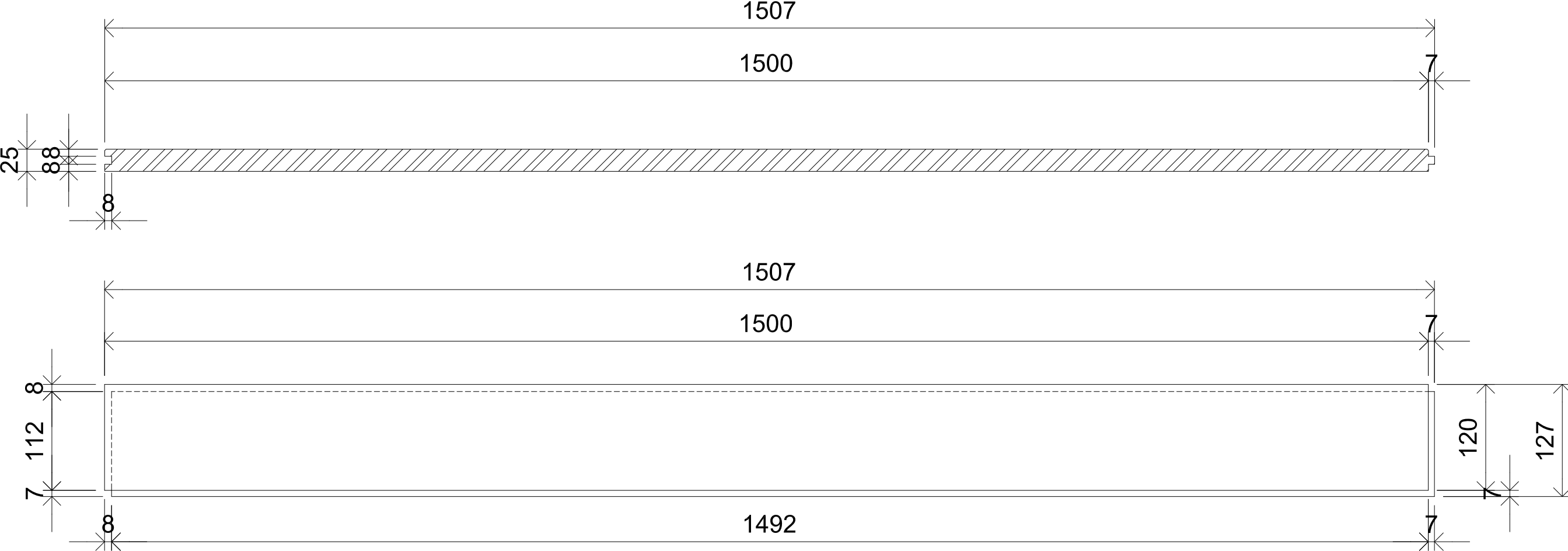
COUPE LONG
