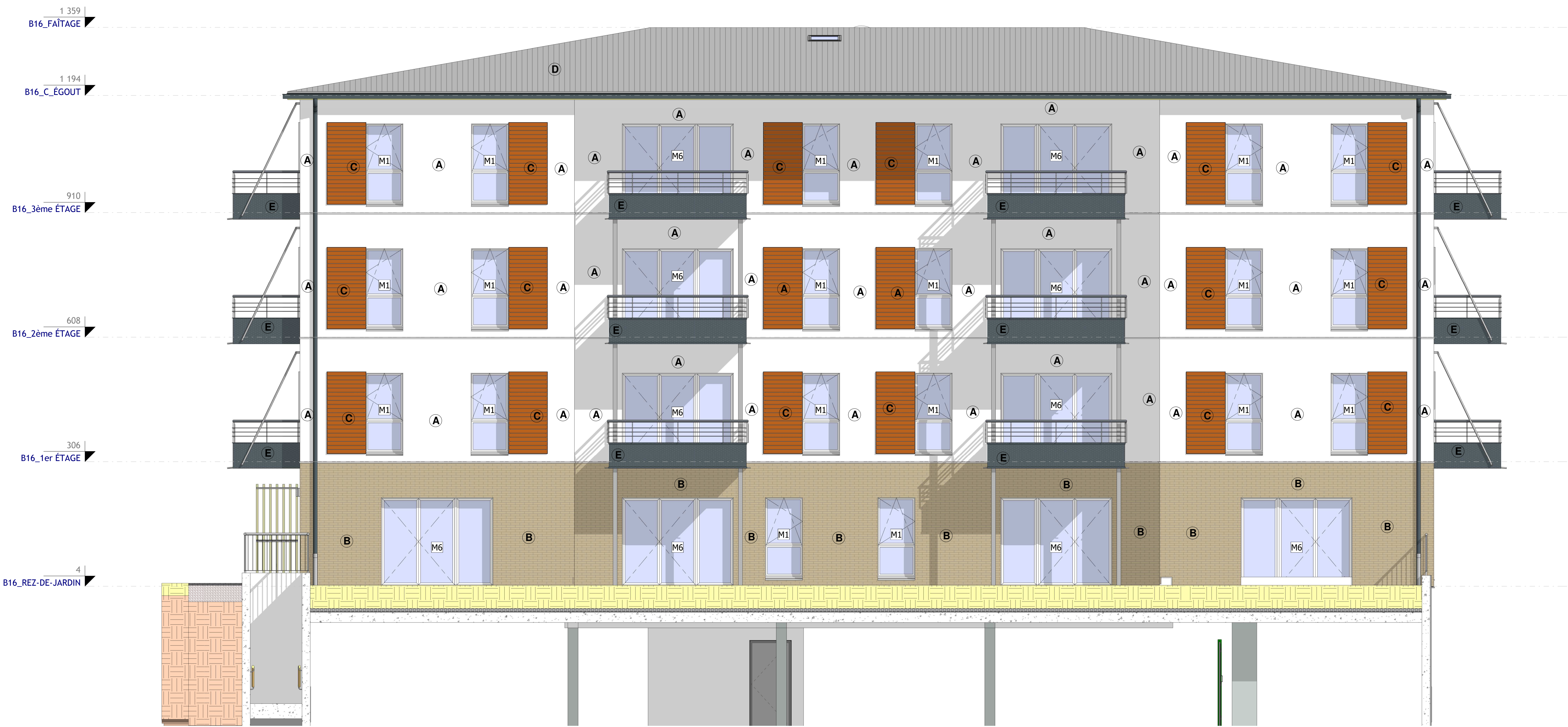
2- B16 - Élévation SUD 1 : 50
