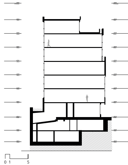
Coupe 5 - EXISTANT
