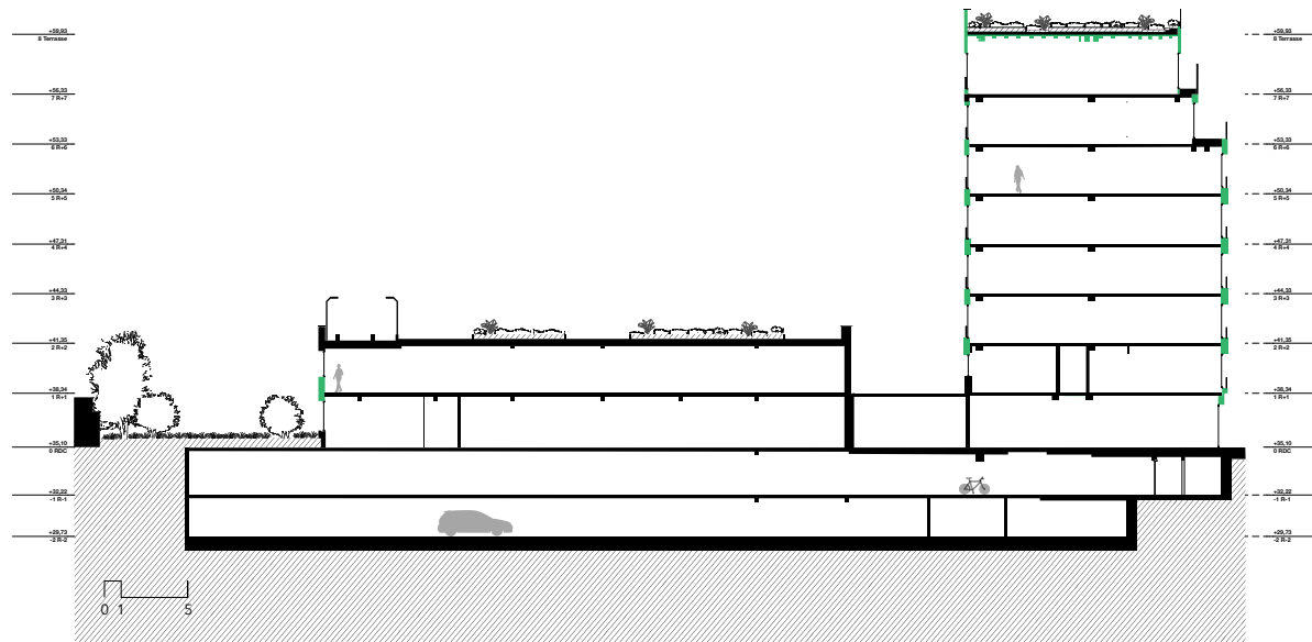
Coupe 2 - PROJET
