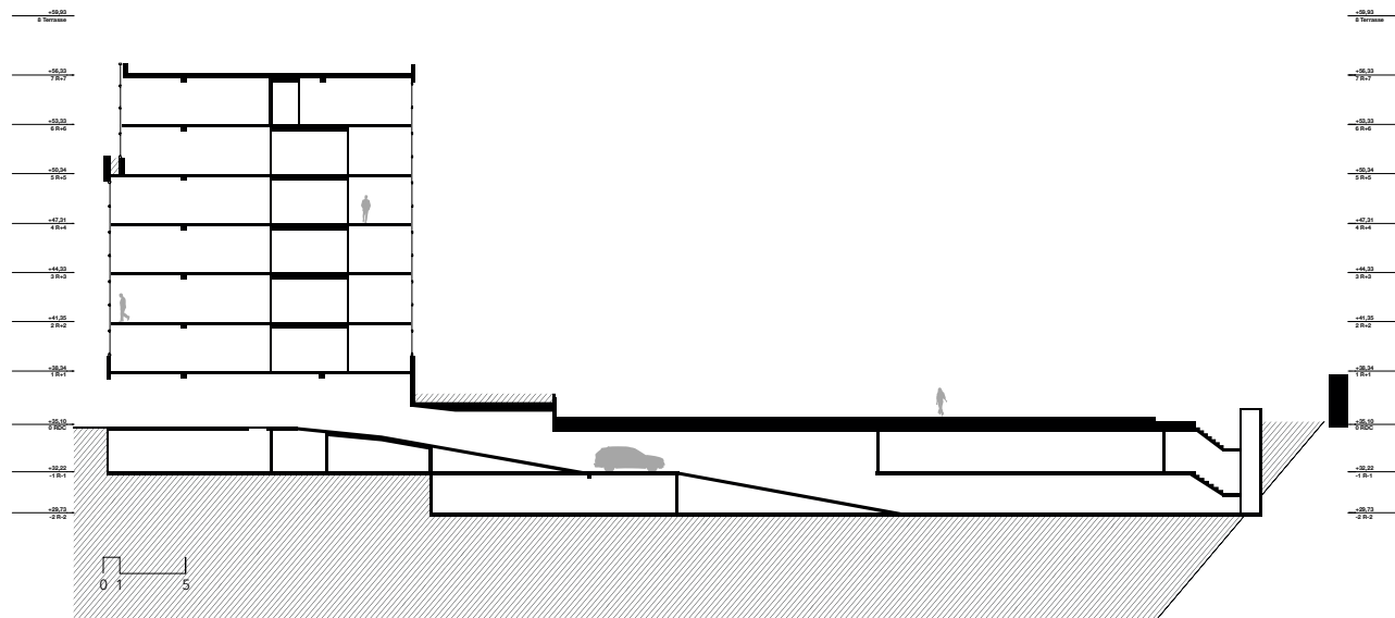
Coupe 1 - EXISTANT
