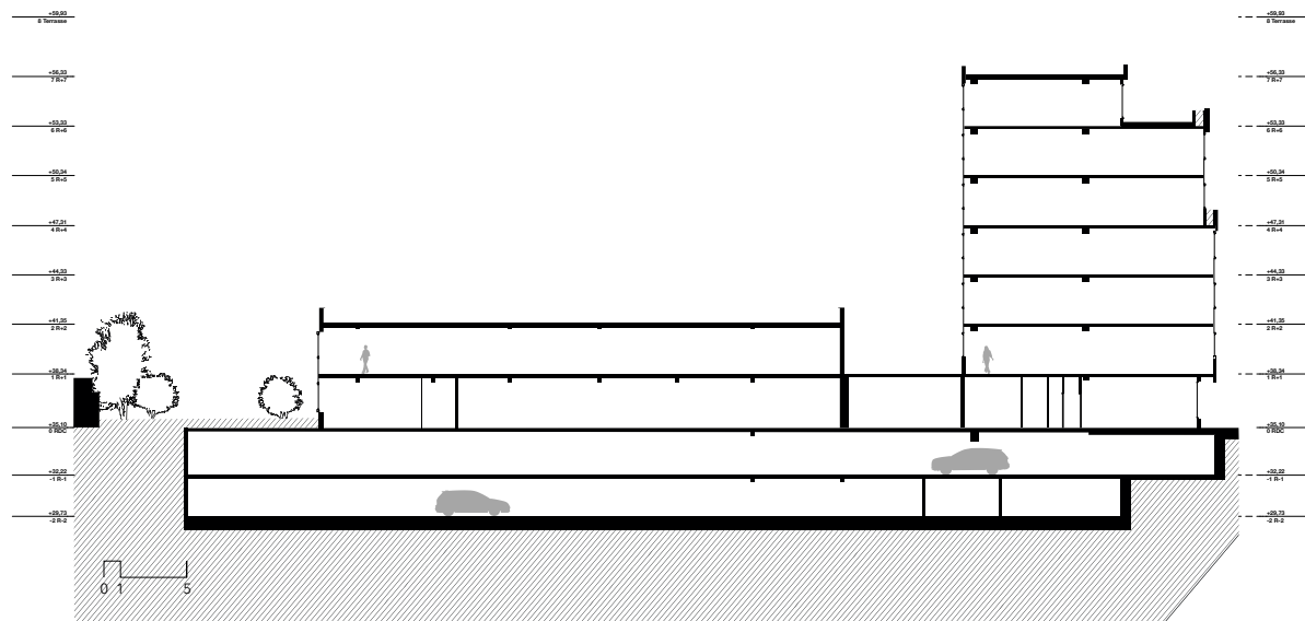
Coupe 2 - EXISTANT
