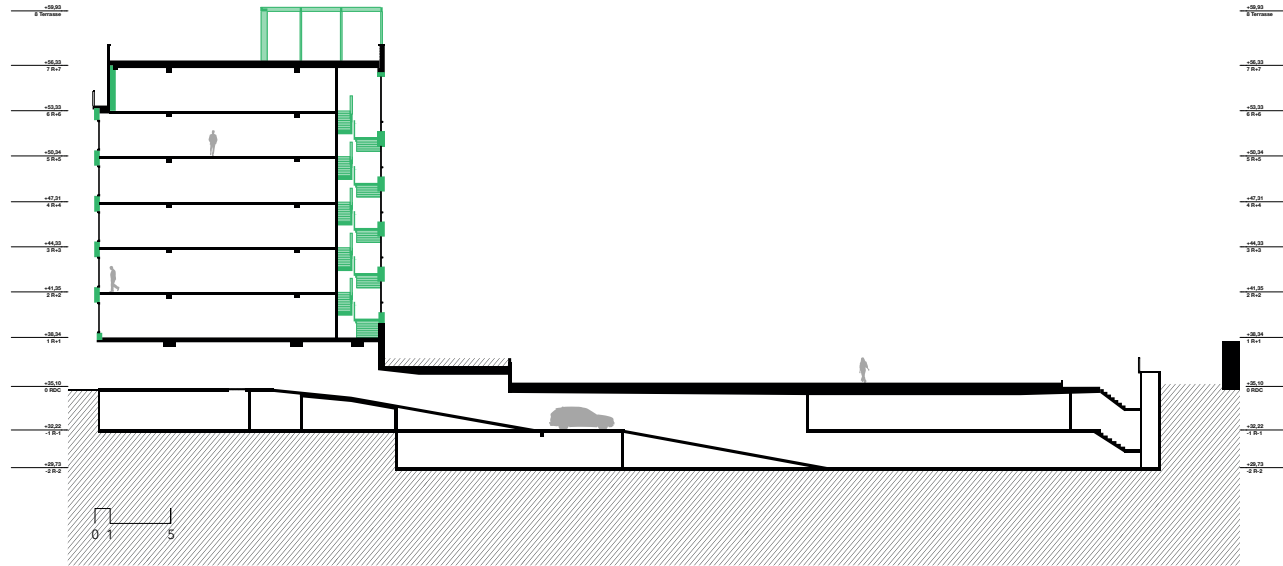
Coupe 1 - PROJET
