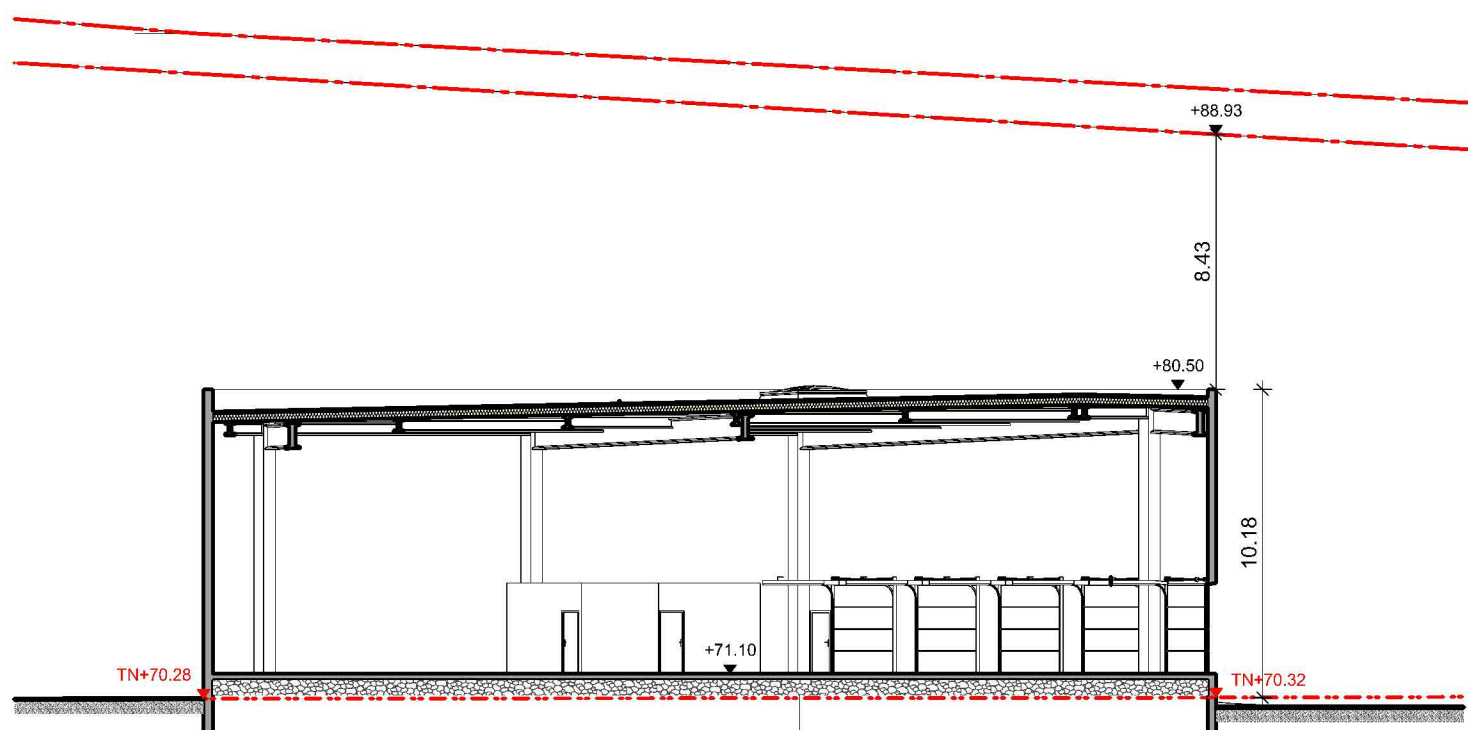
Coupe sur bâtiment 2 sous la ligne THT (Hauteur relevé par géomètre) Ech 1/250
