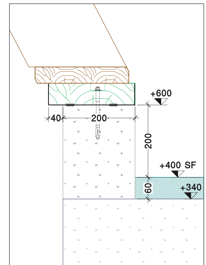
Détail de principe du relevé béton
