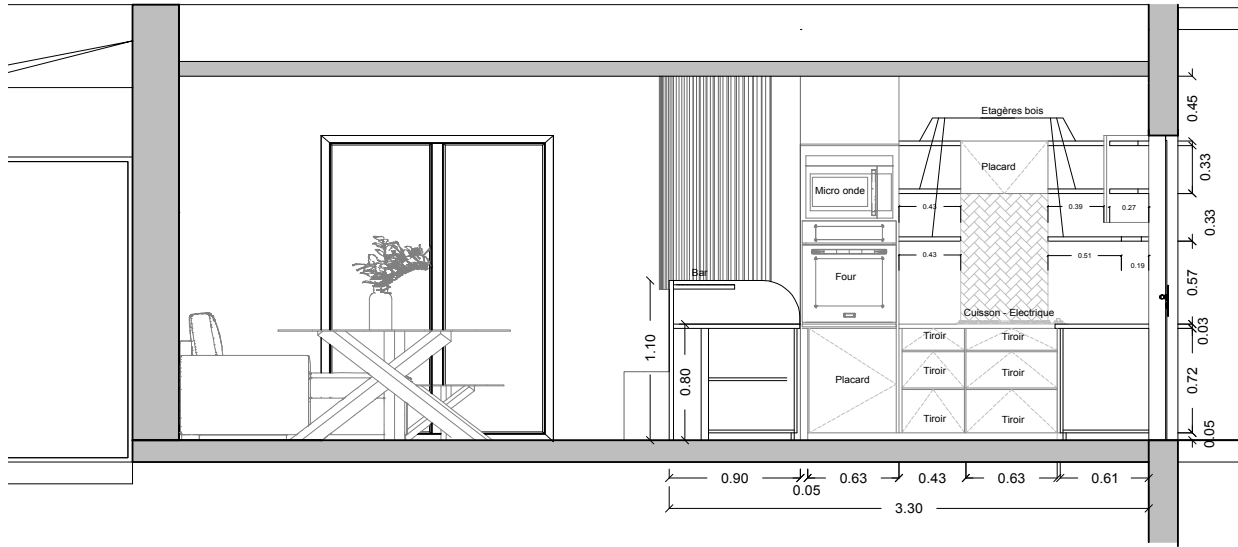
COUPE AA'
