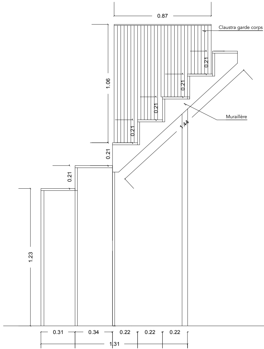
Élévation arrière de l'escalier
