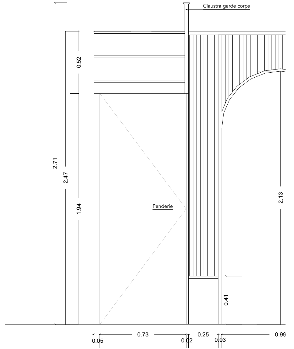
Élévation gauche de l'escalier
