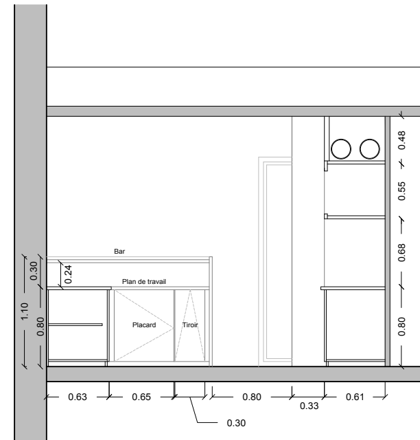
COUPE CC'
