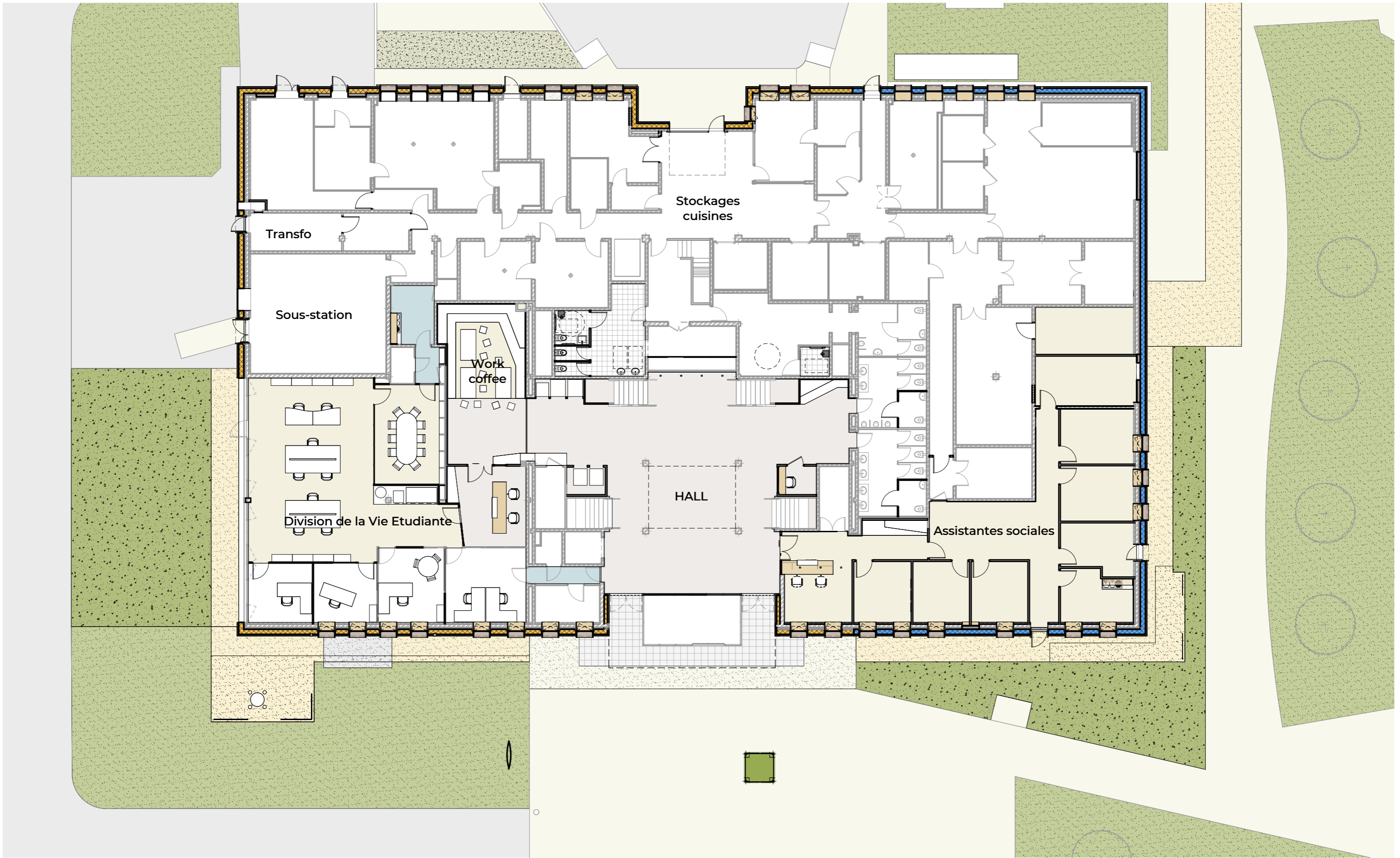
REZ-DE-CHAUSSEE PROJET
