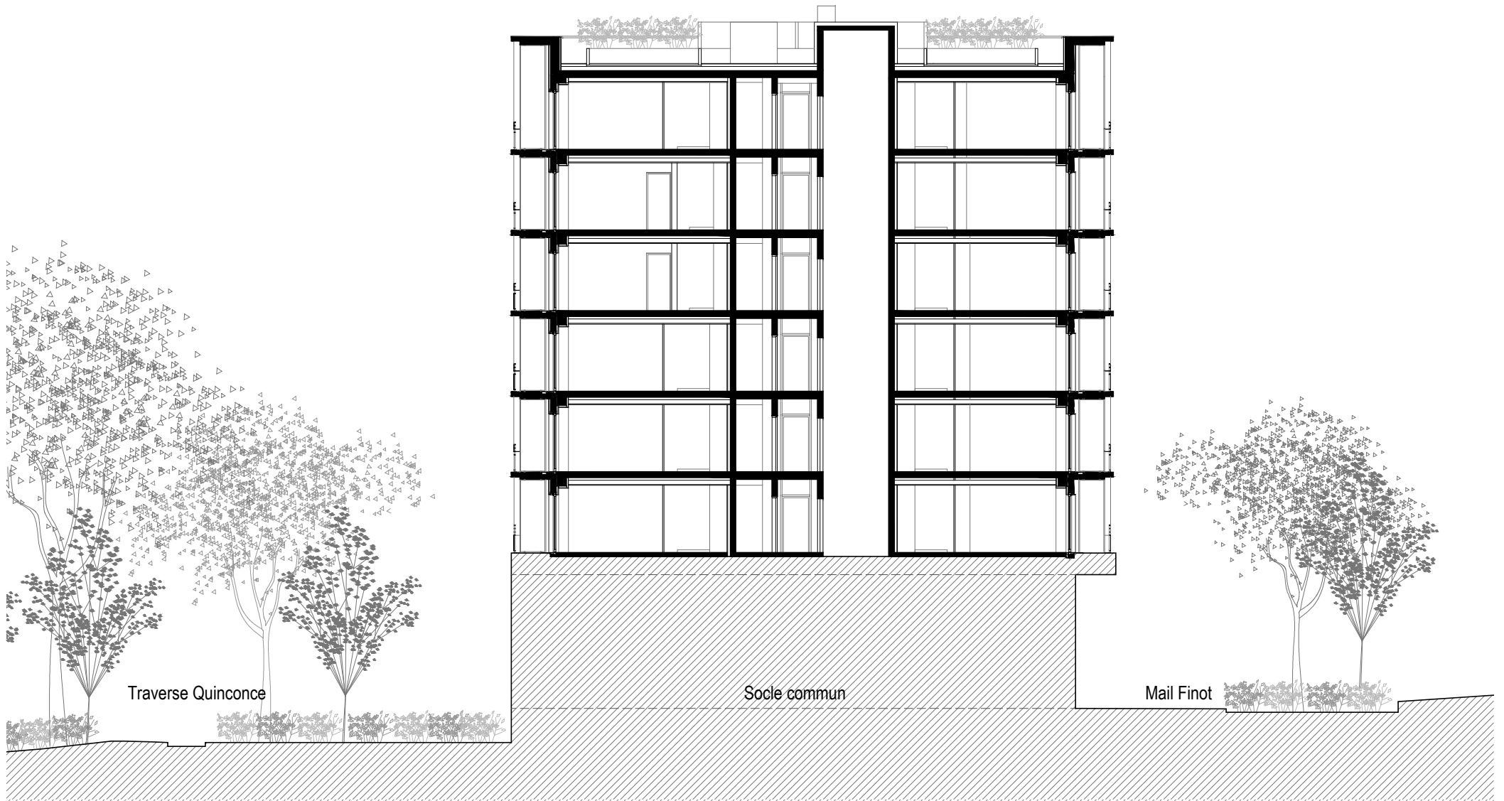
Coupe transversale sur traverse Quinconce et Mail Finot
