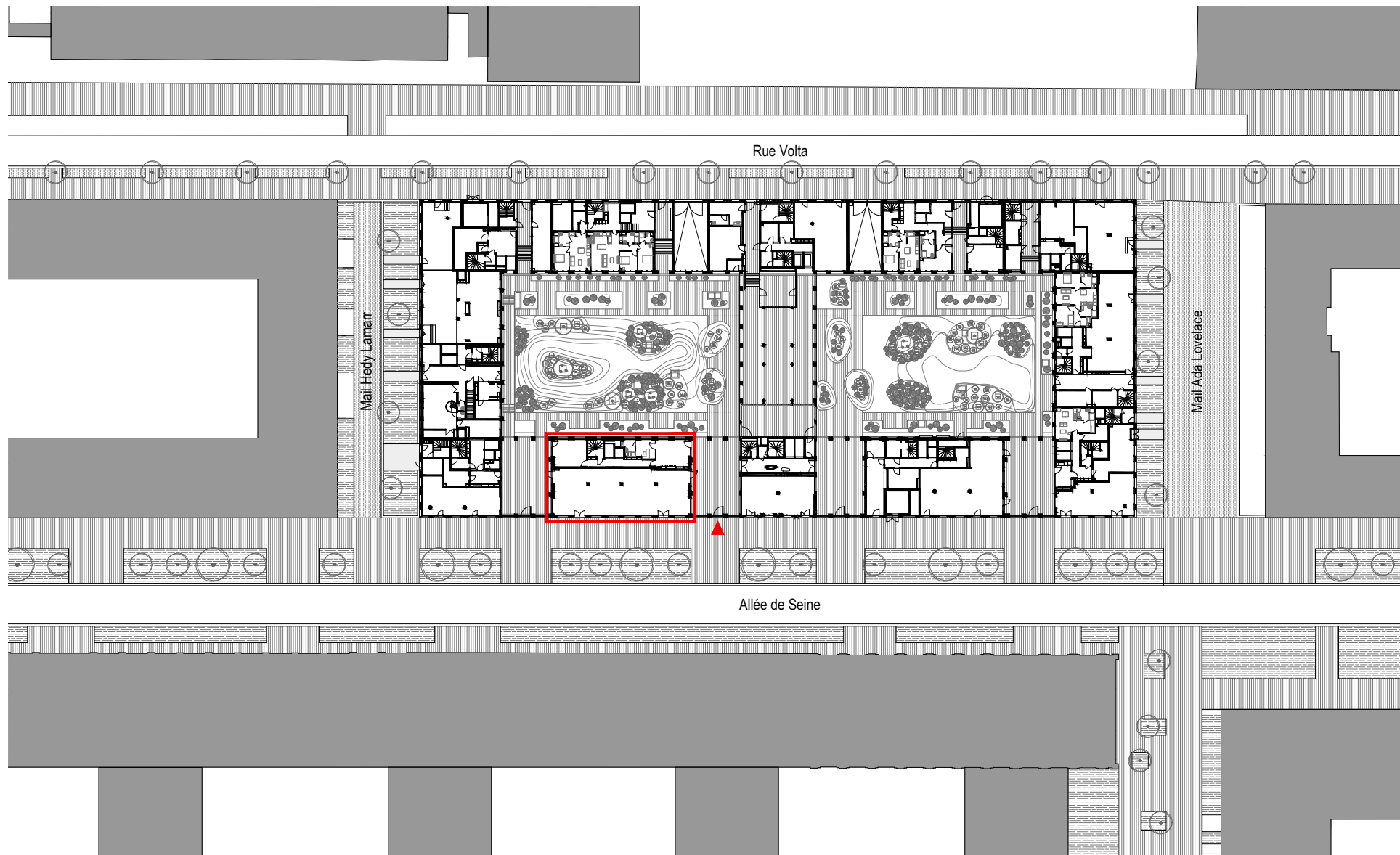
Plan rez de chaussée îlot A2
