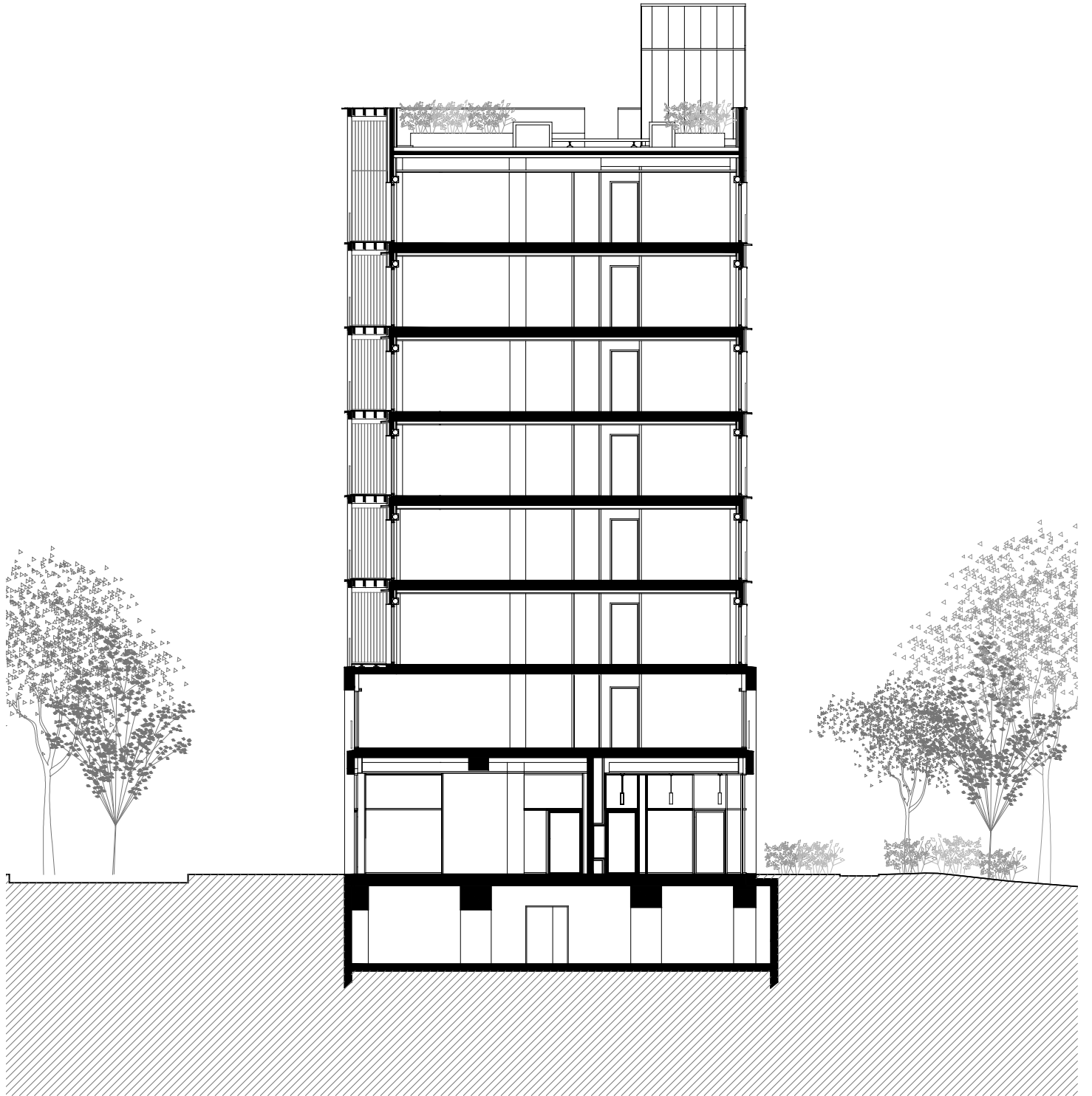
Coupe transversale sur rue et cour
