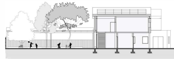
COUPE TRANSVERSALE
