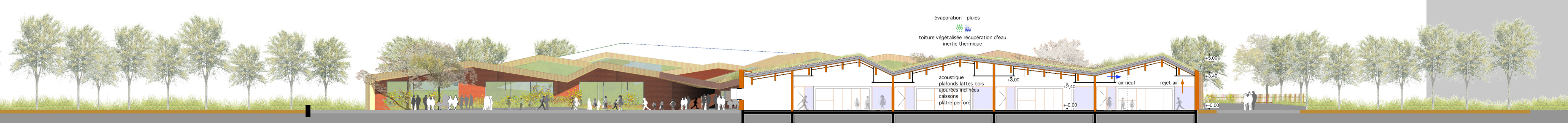
COUPE longitudinale salles de classe élémentaire échelle 1/200e
