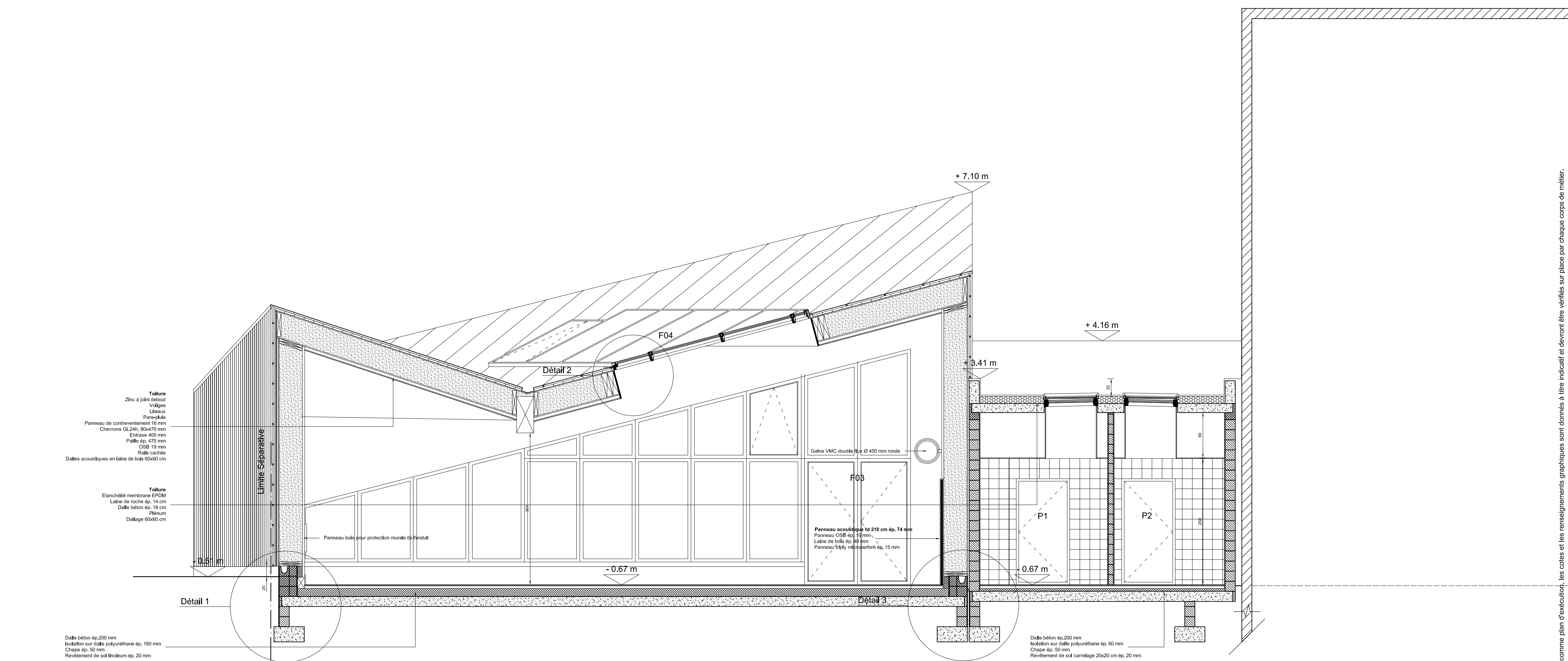
Coupe ZZ Projet
