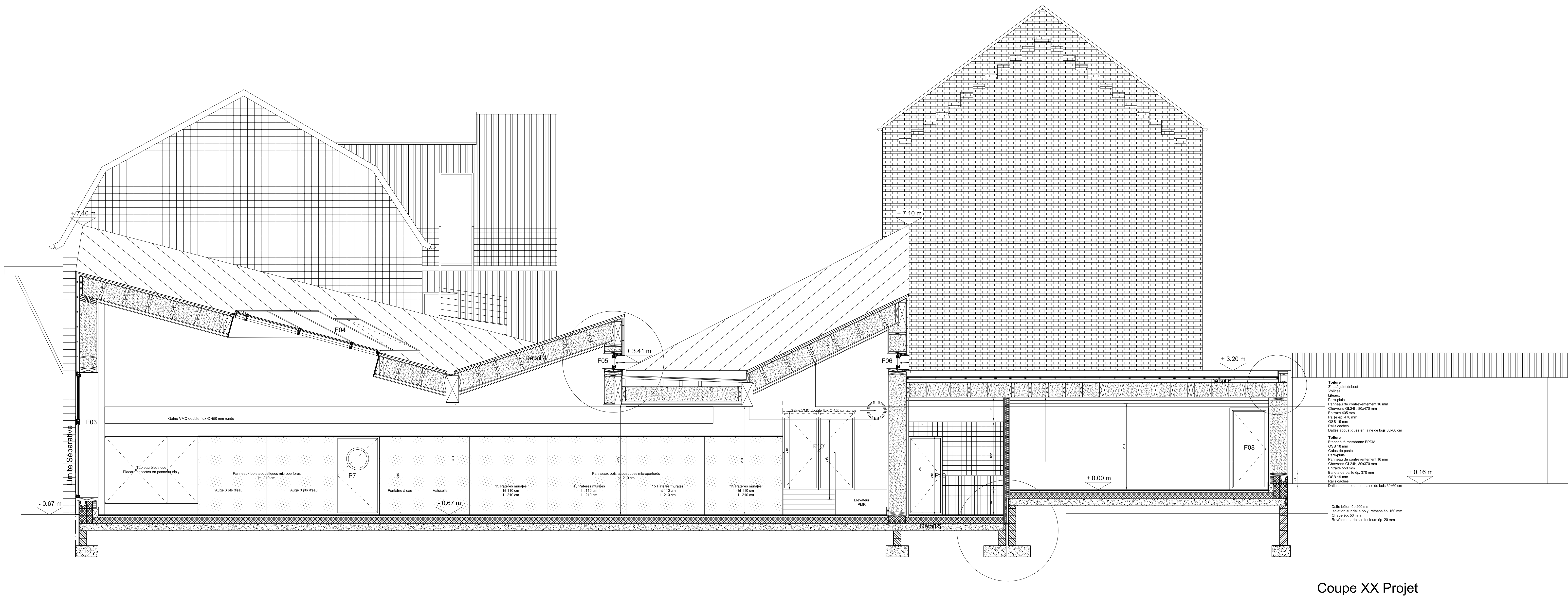
Coupe XX Projet
