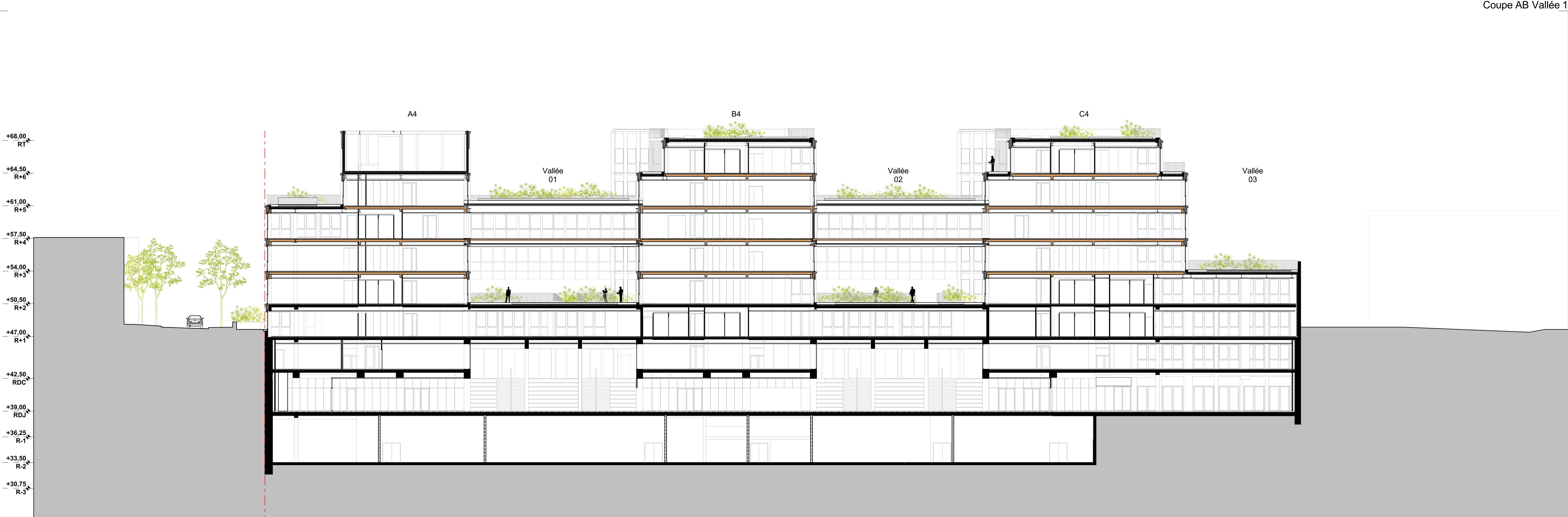
Coupe AB Vallée 1
