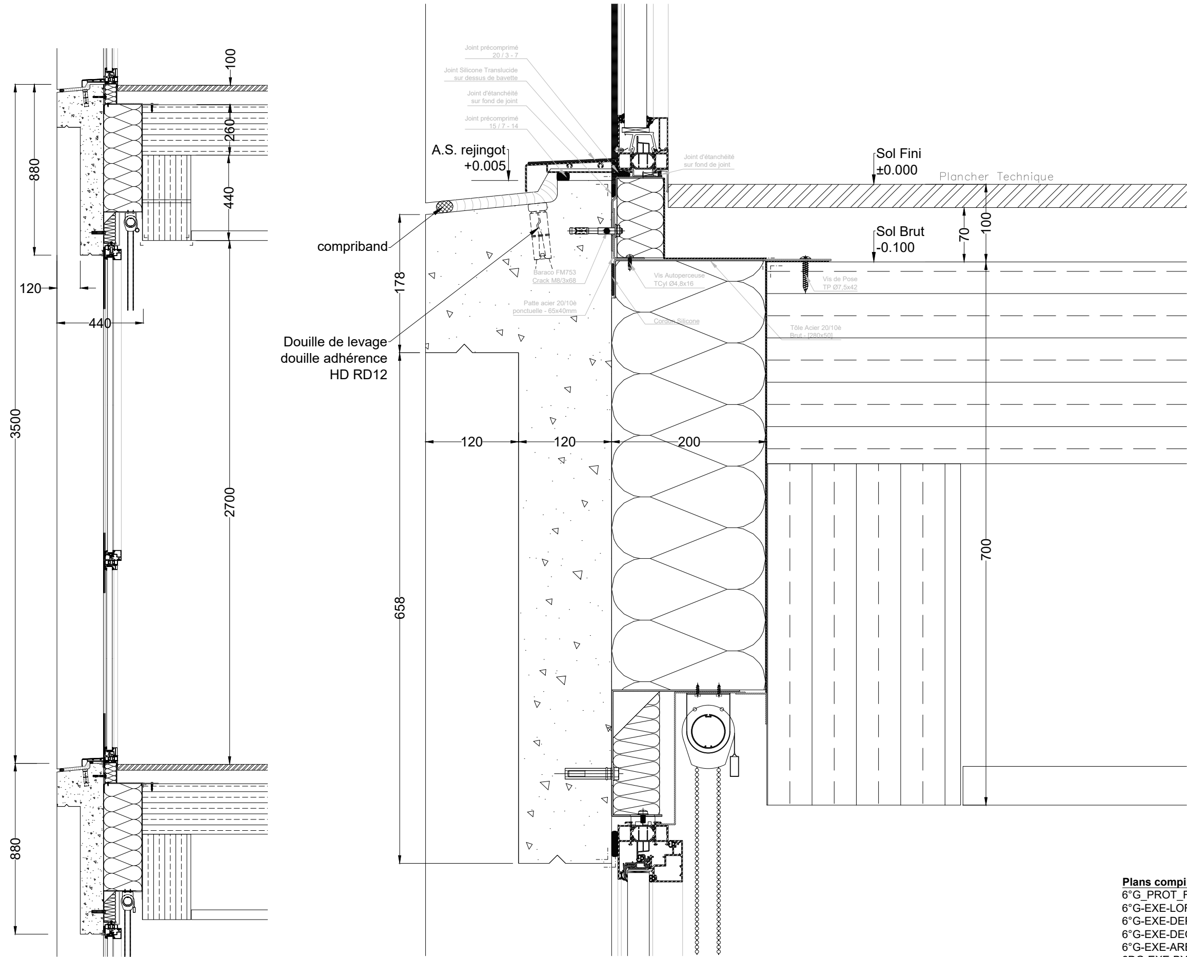
Coupe 1
