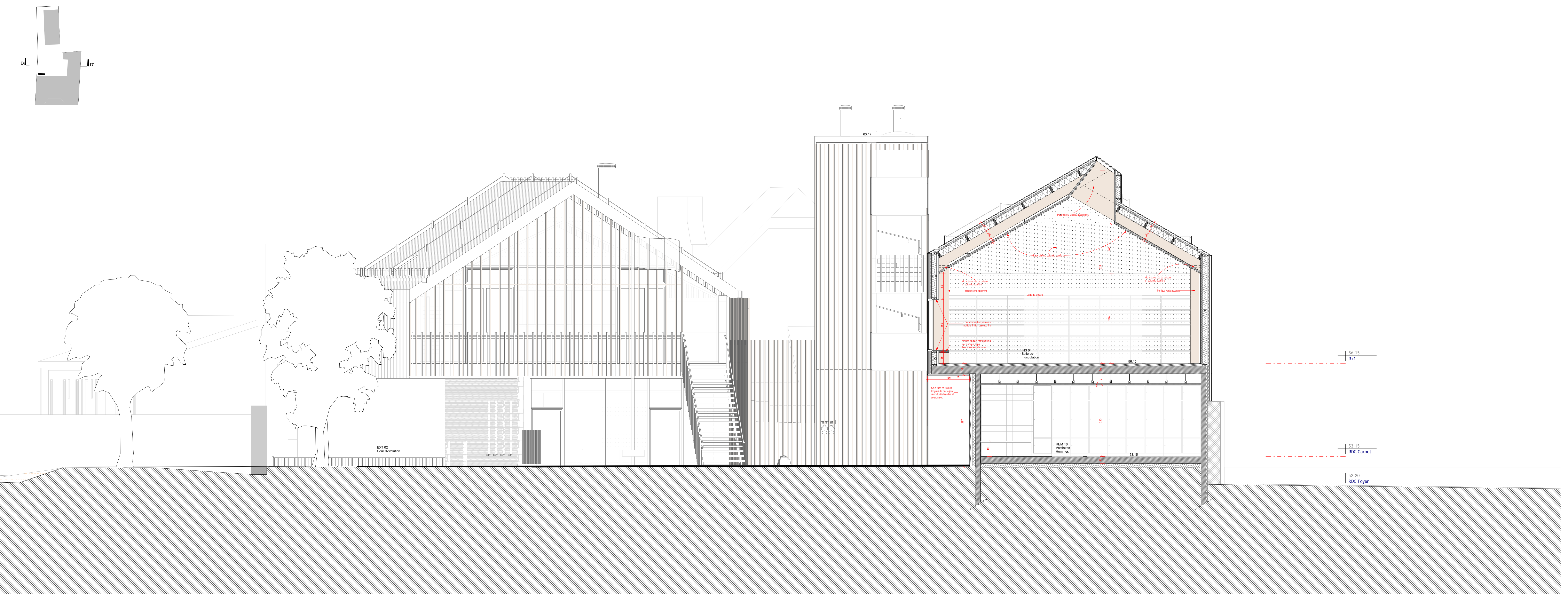
COUPE TRANSVERSALE - GYMNASE - ÉCHELLE 1:50
