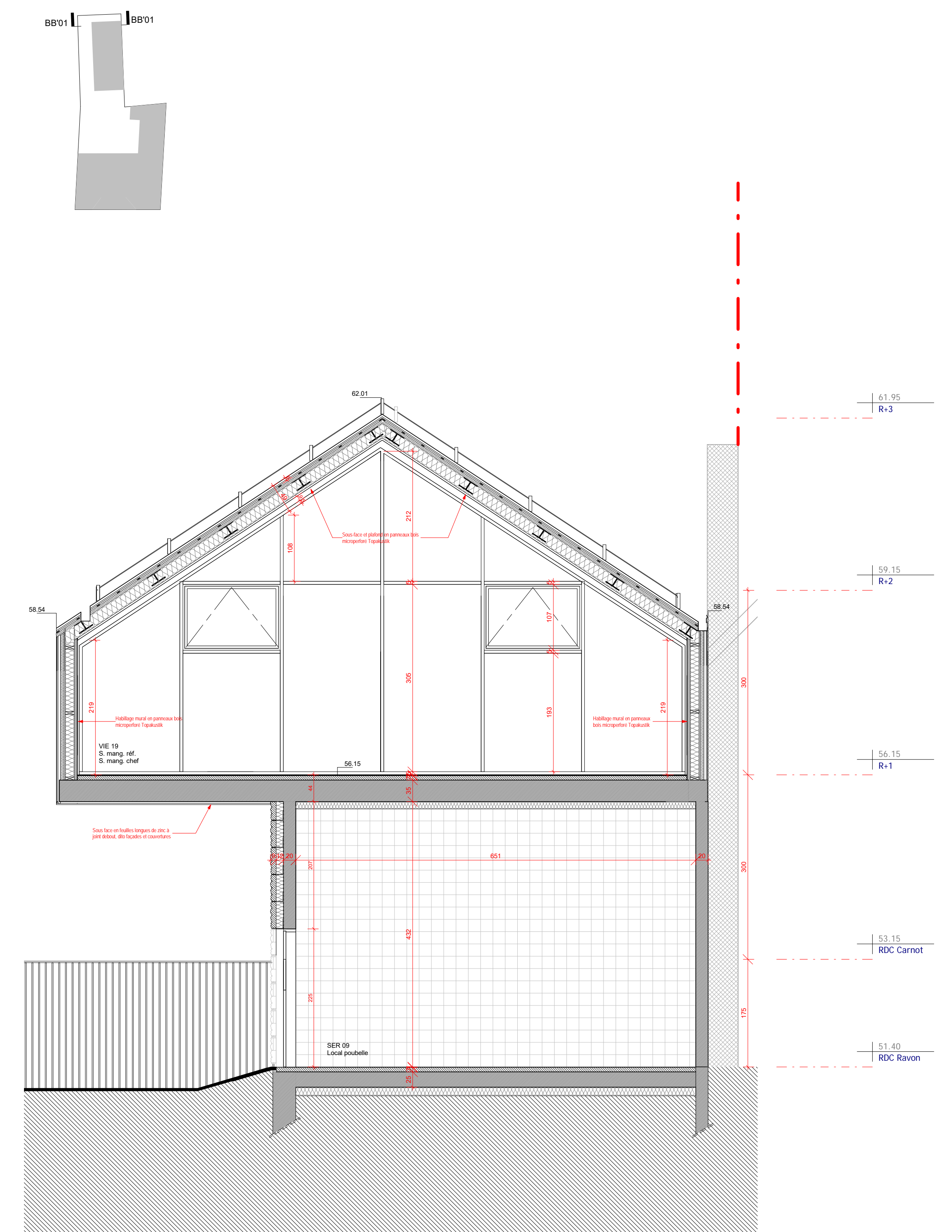
COUPE TRANSVERSALE - REFECTOIRE OFFICERS- ÉCHELLE 1:50
