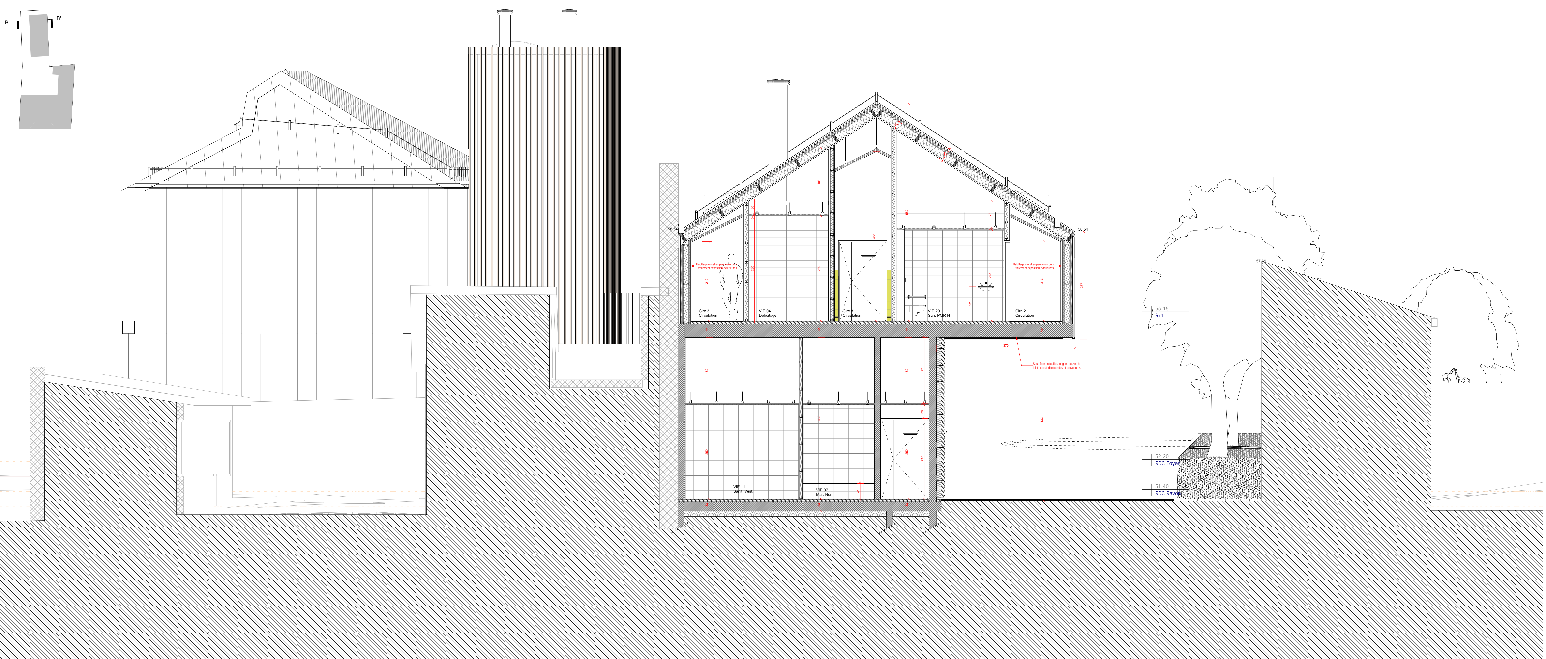
COUPE TRANSVERSALE - CUISINE - ÉCHELLE 1:50
