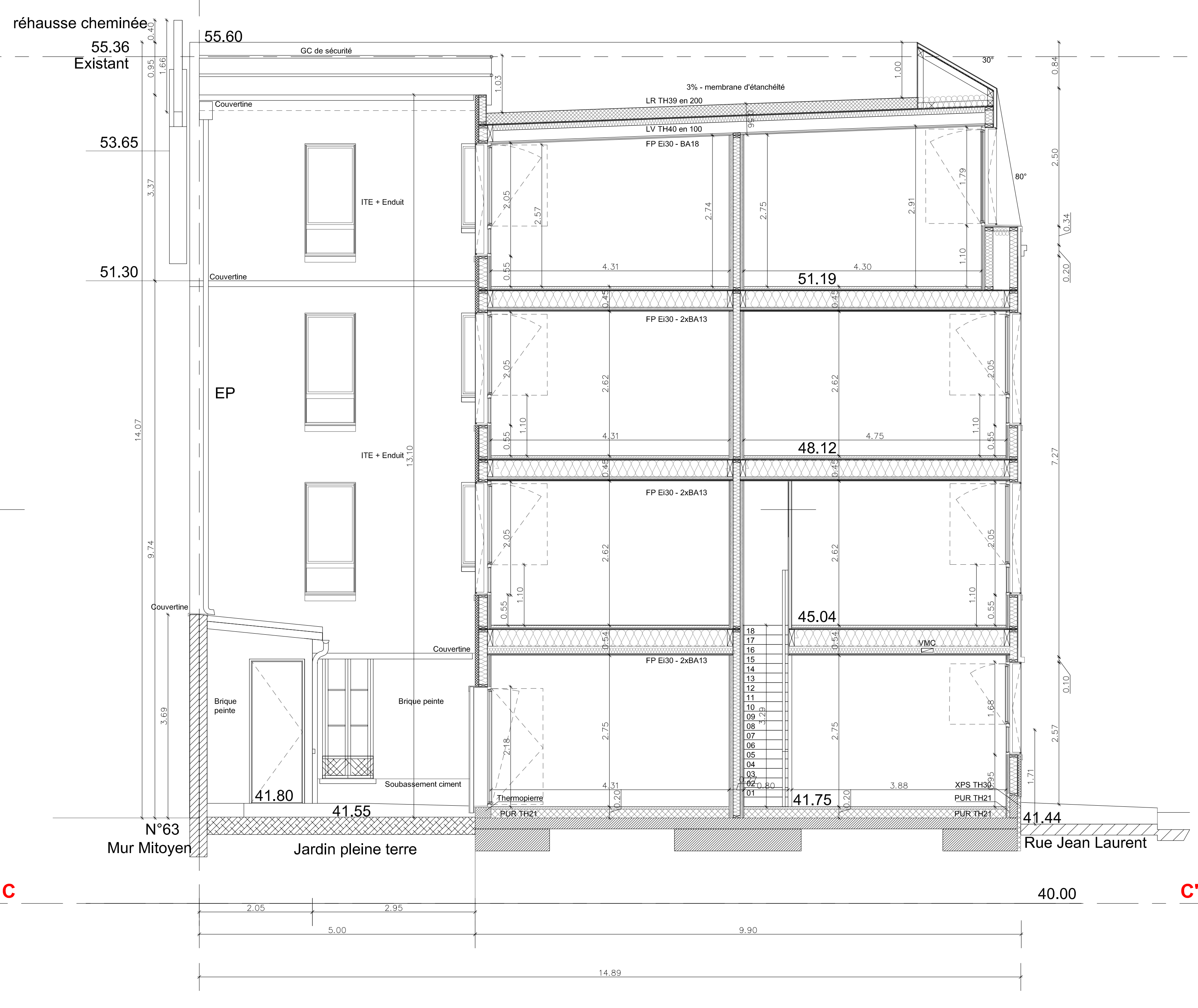
ELEVATION COUR NORD - COUPE SUR EXTENSION RUE J.LAURENT
