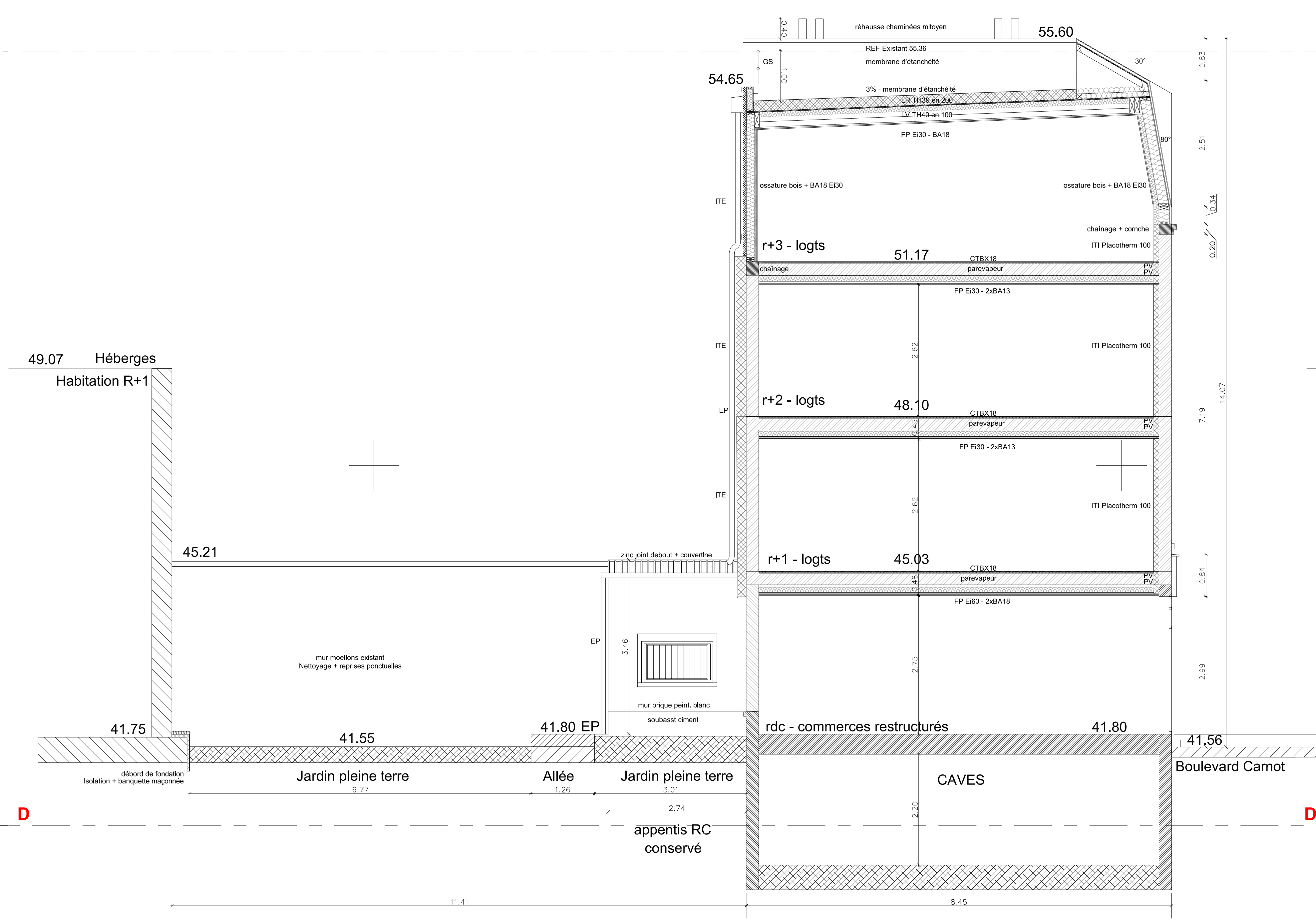
ELEVATION COUR OUEST - COUPE SUR EXISTANT BD CARNOT
