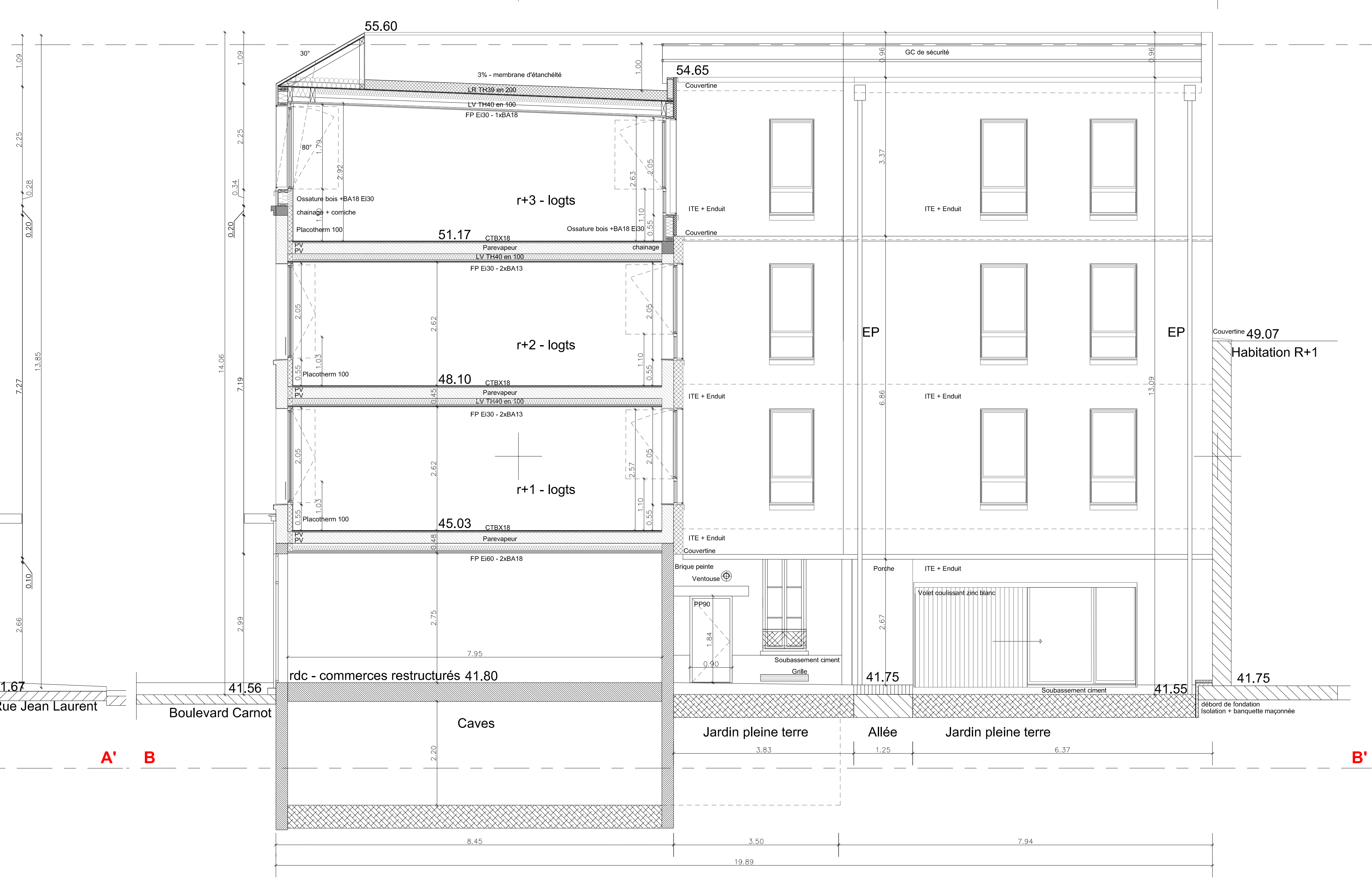
ELEVATION COUR NORD - COUPE SUR EXISTANT RUE J.LAURENT
