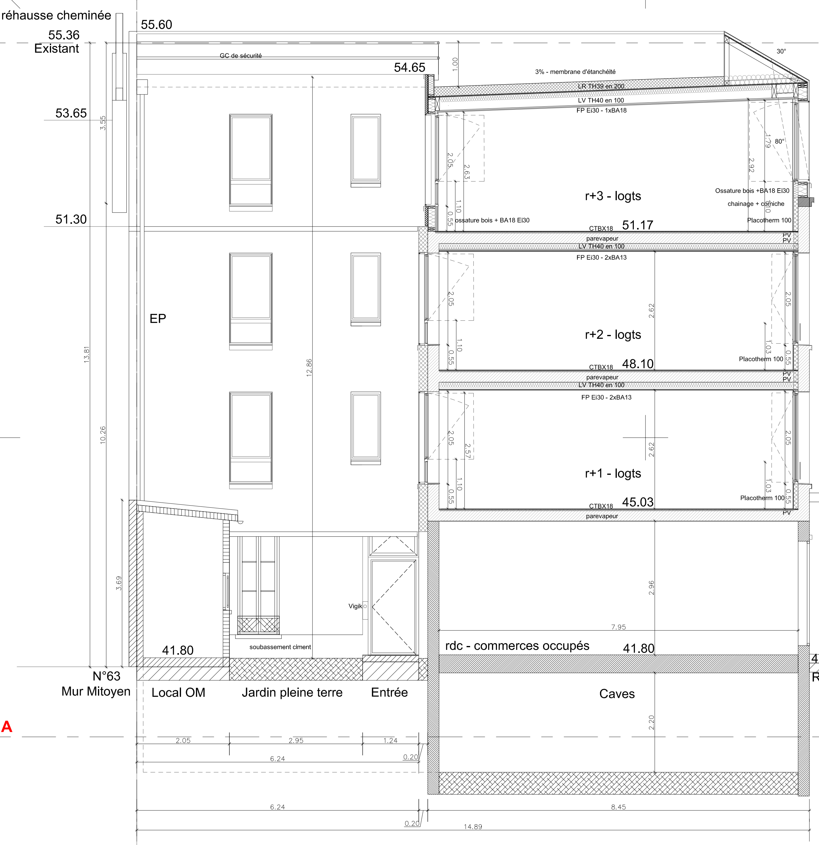
ELEVATION COUR NORD - COUPE SUR EXISTANT RUE J.LAURENT
