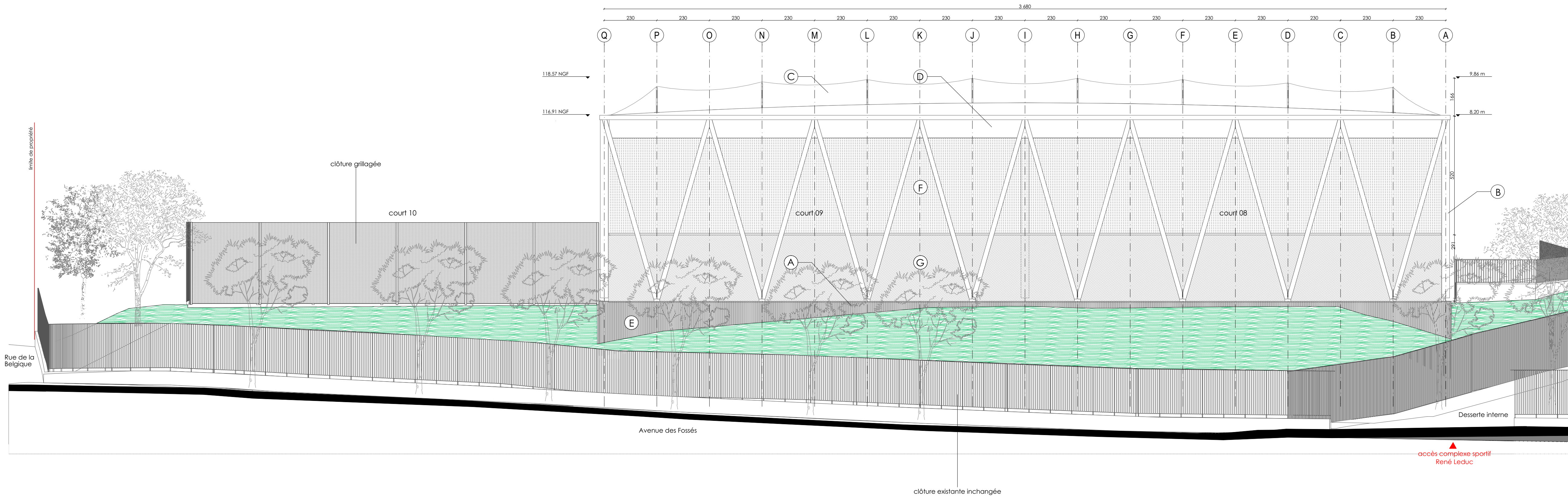
élévation nord
