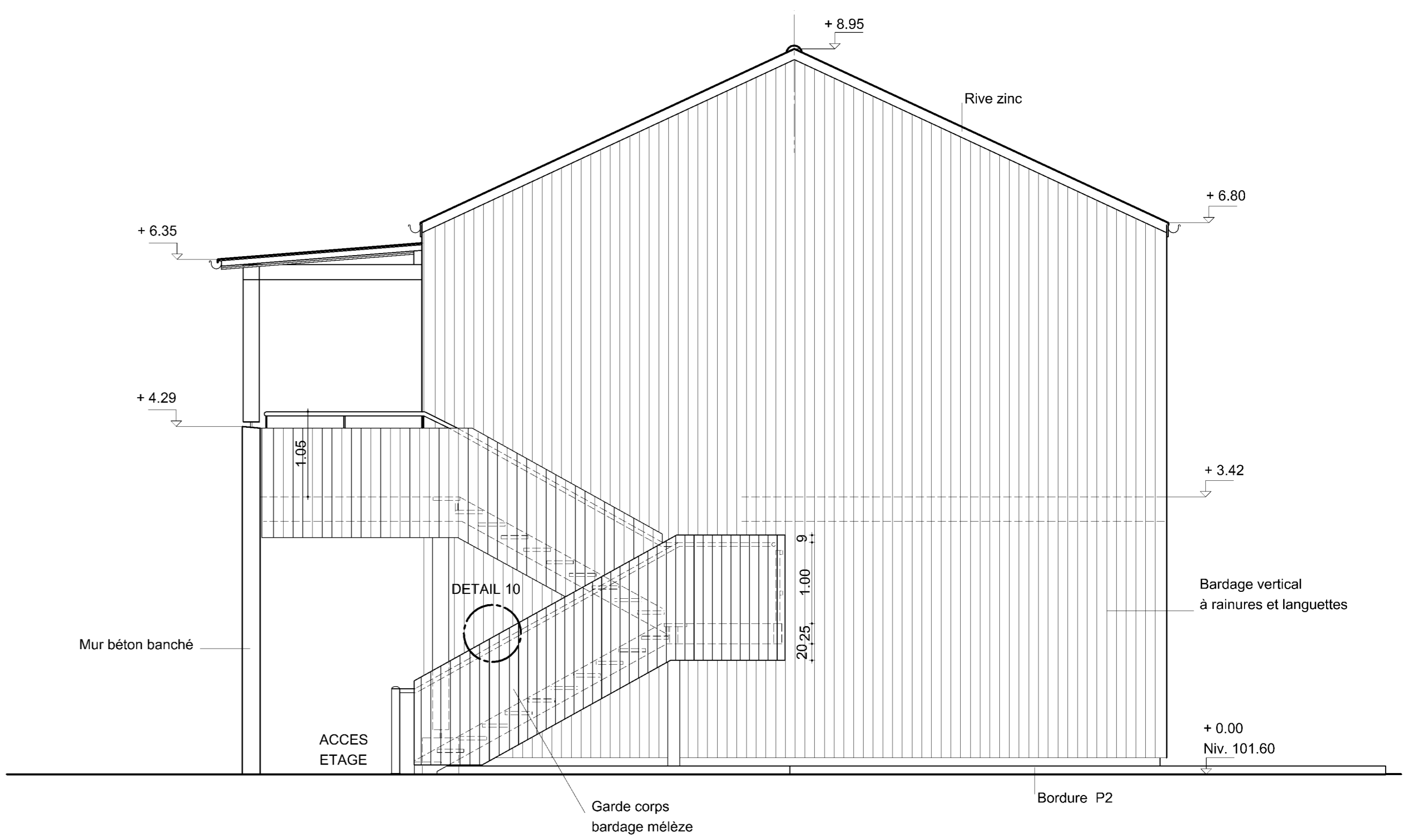
FACADE EST
