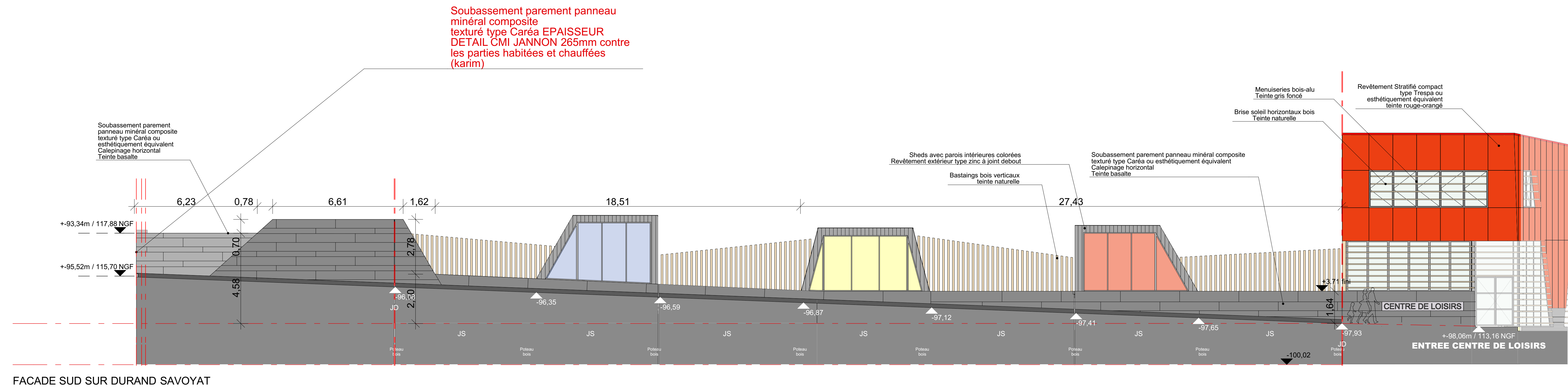
FAÇADE SUD SUR DURAND SAVOYAT
