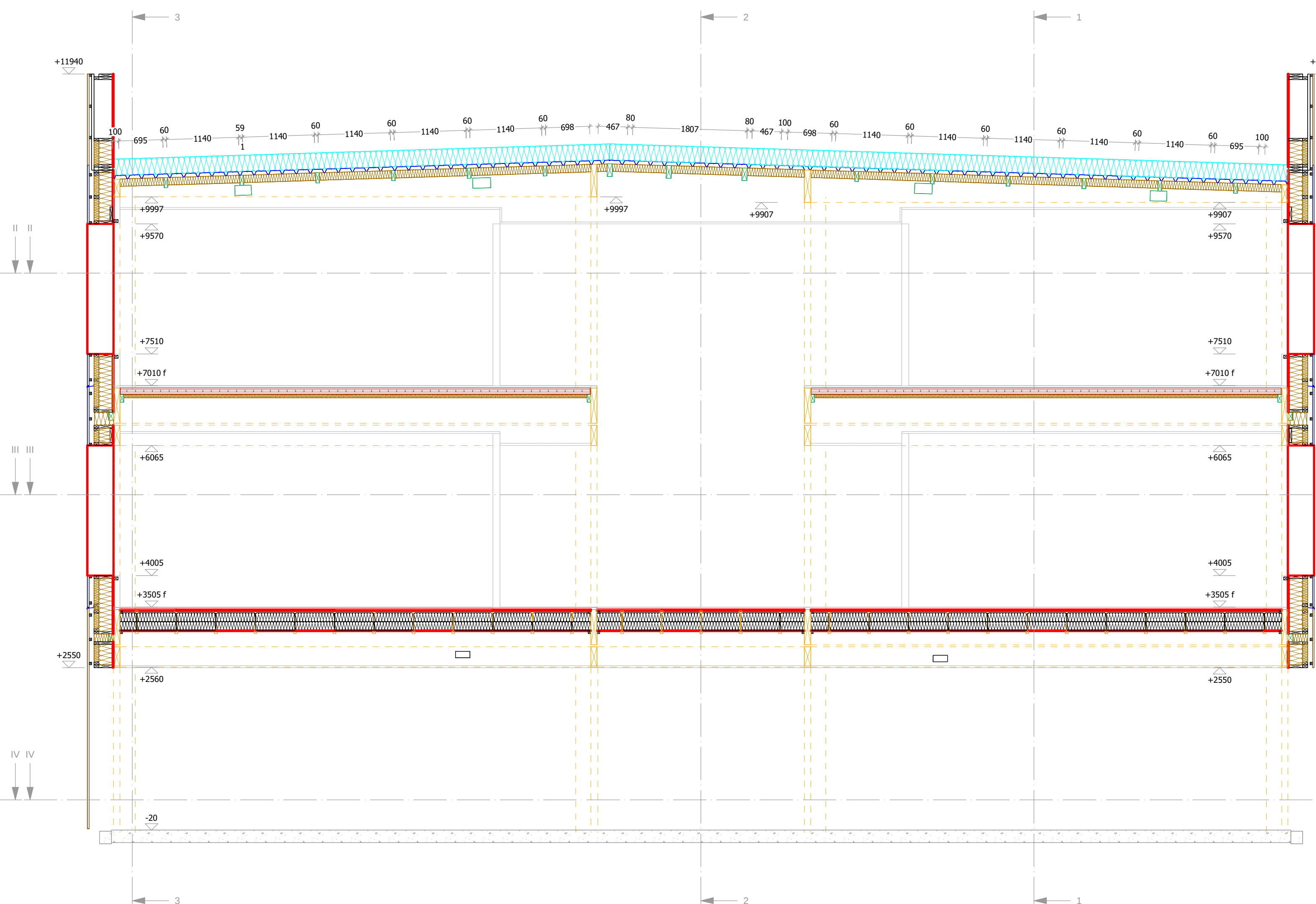
Coupe: A-A Echelle: 1:50
