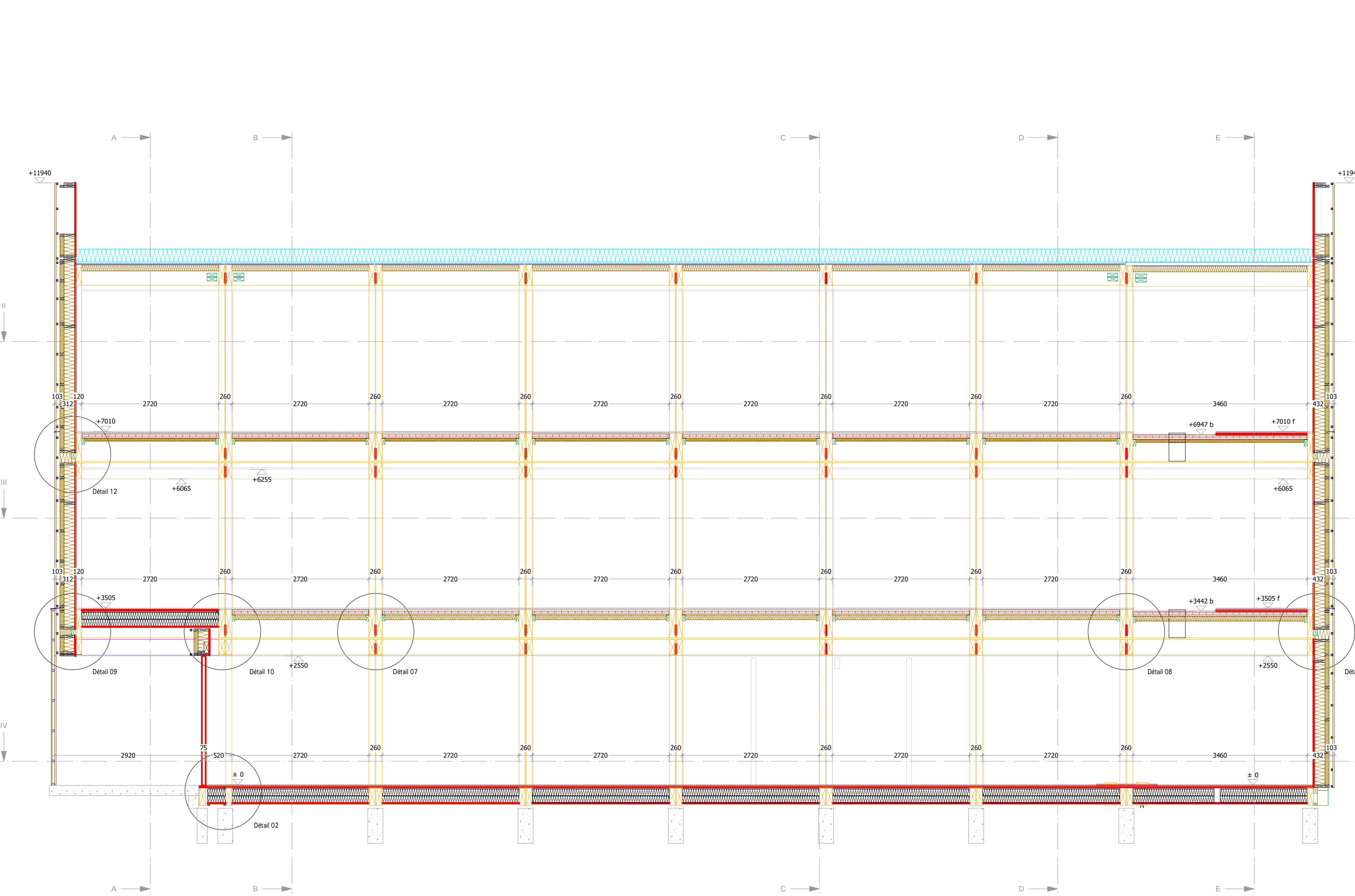
Coupe: 1-1 Echelle: 1:50
