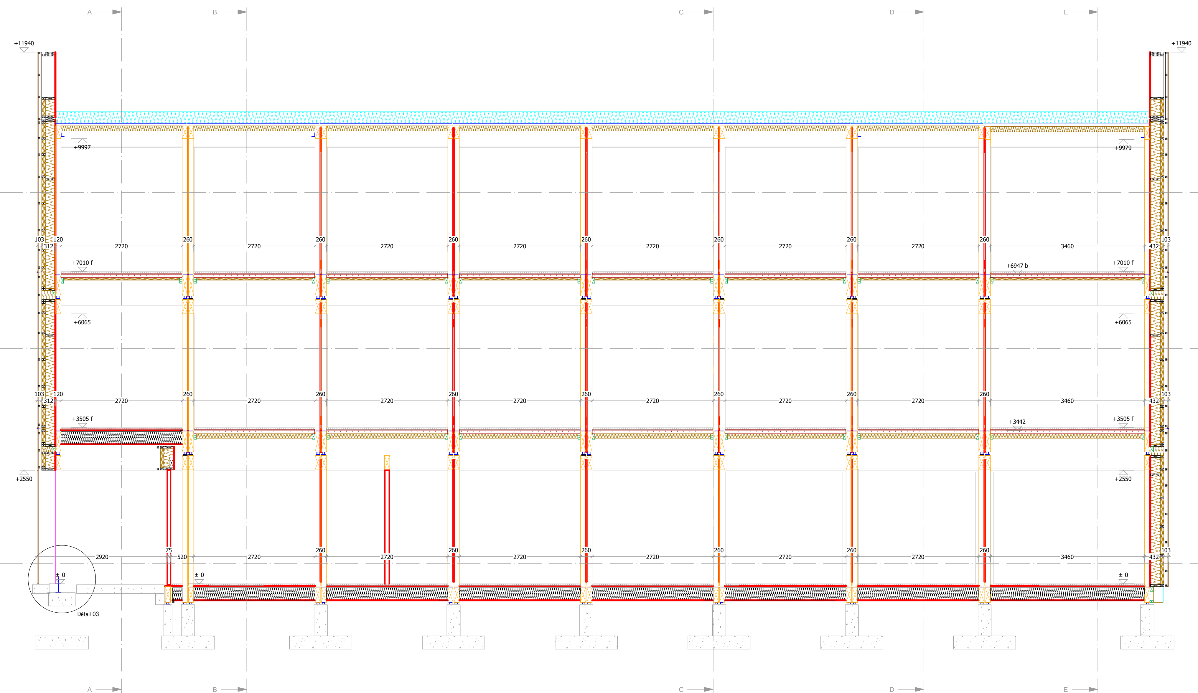
Coupe: 3-3 Echelle: 1:50
